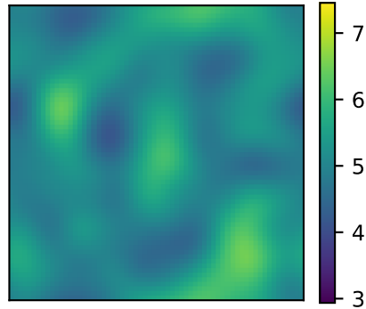
posterior mean
