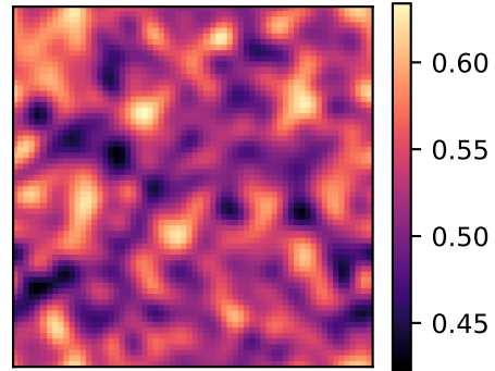
posterior SD
