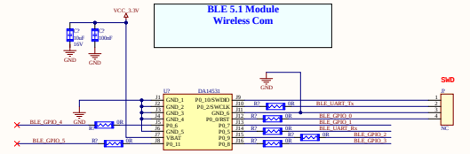
BLE 5.1 Module
