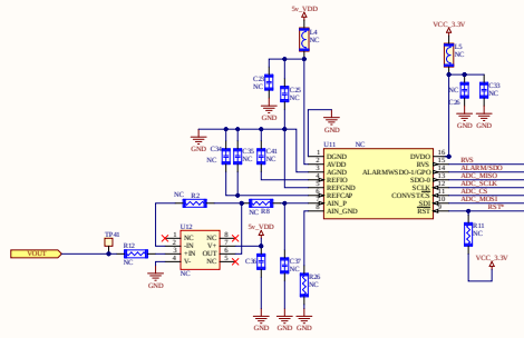
ANA_OUT_ADC - Optional
