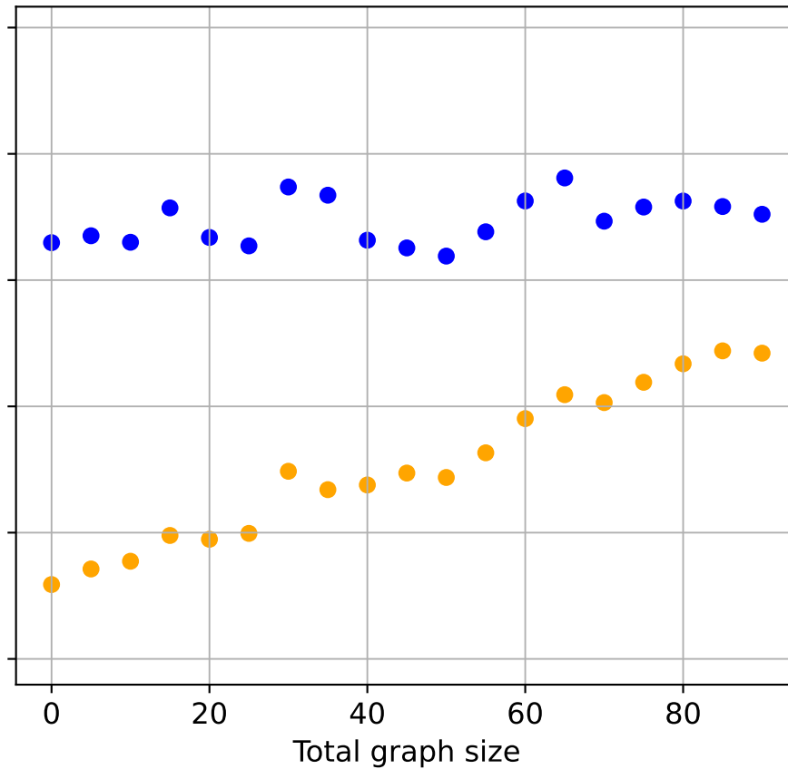
MLP
