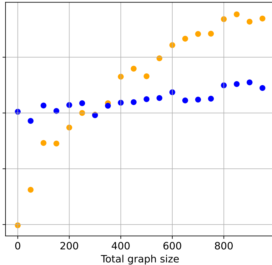
MLP
