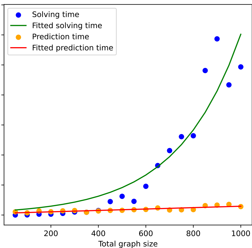
MLP
