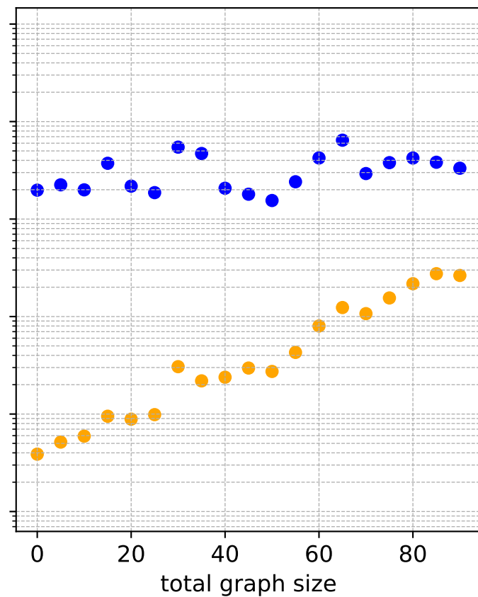
MLP
