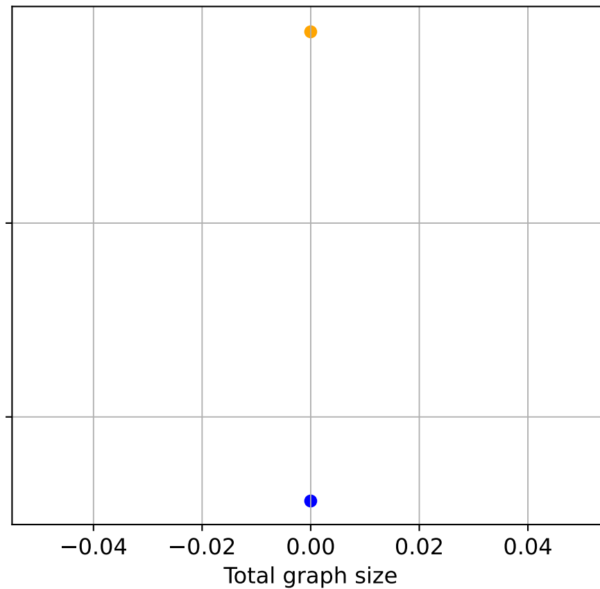
MLP
