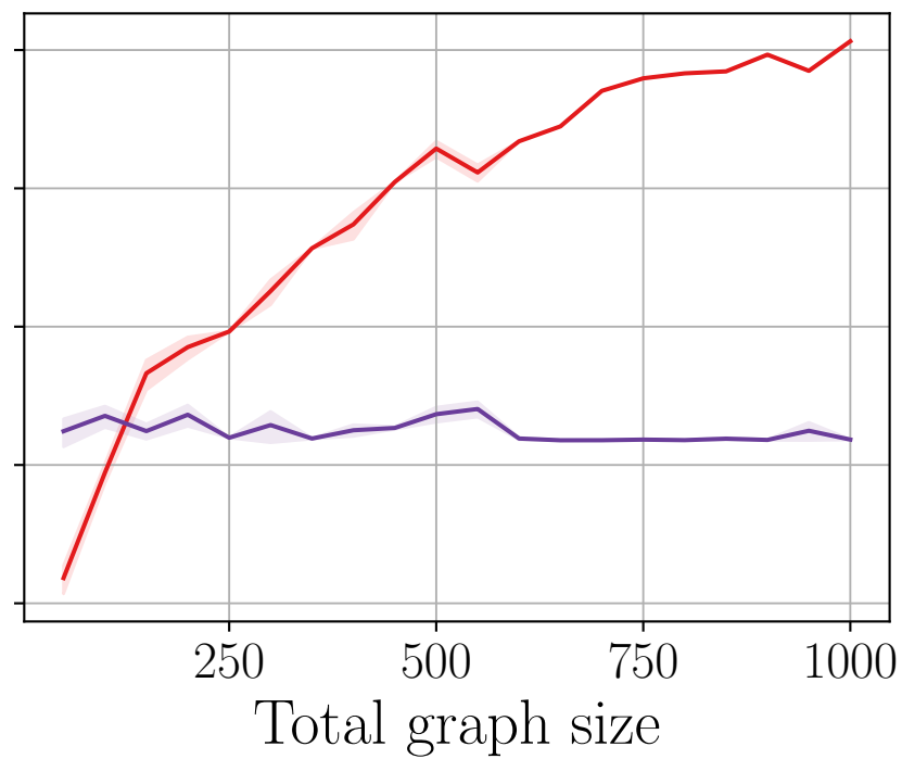
(b) MLP
