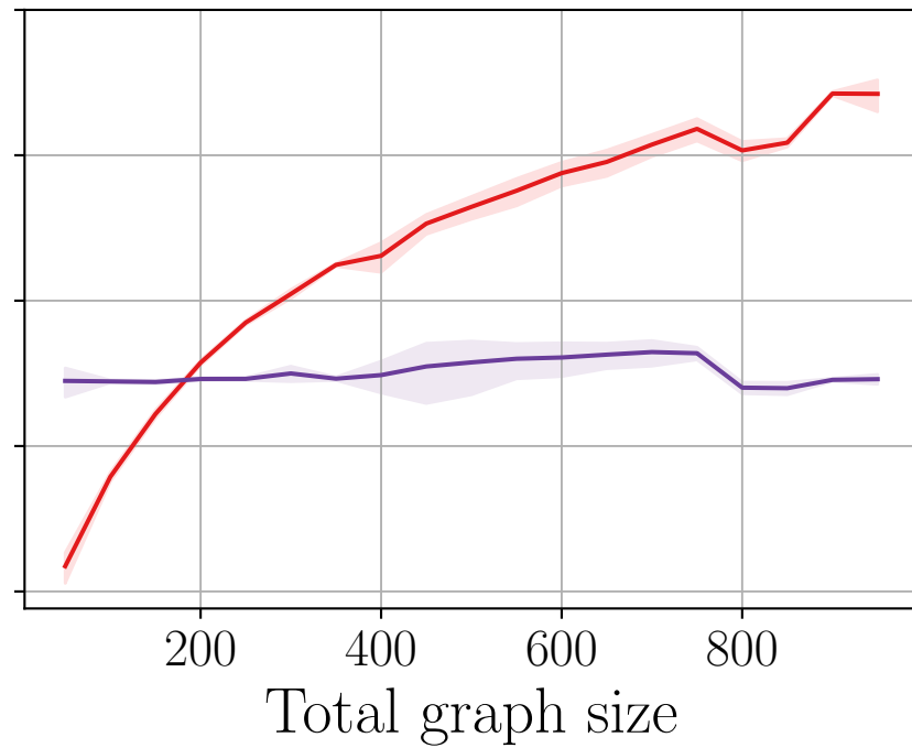
(b) MLP
