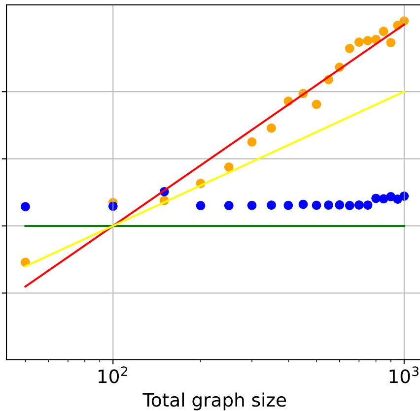
MLP
