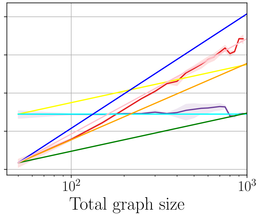
(b) MLP
