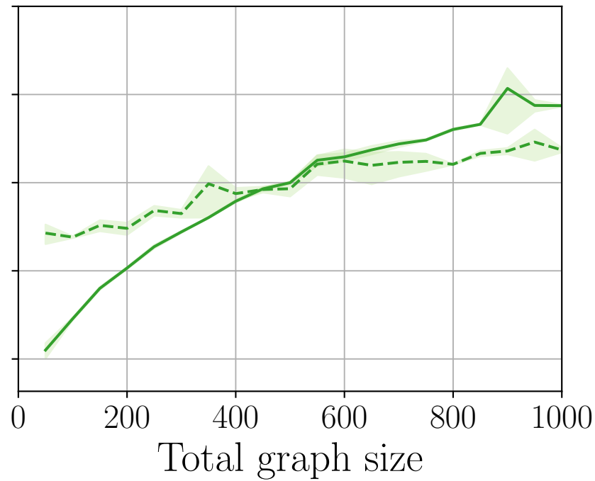
(b) MLP
