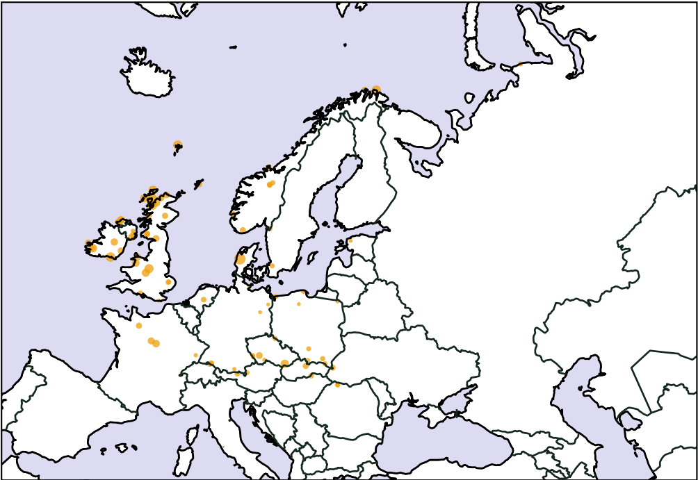
11500-10000 BP
