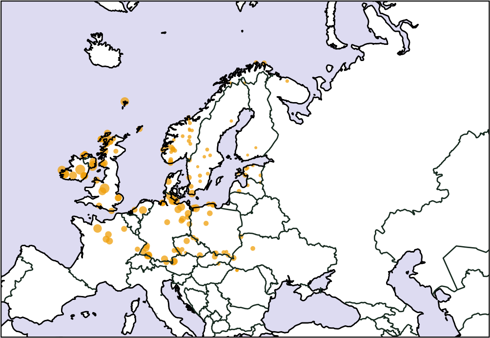
4000-2000 BP
