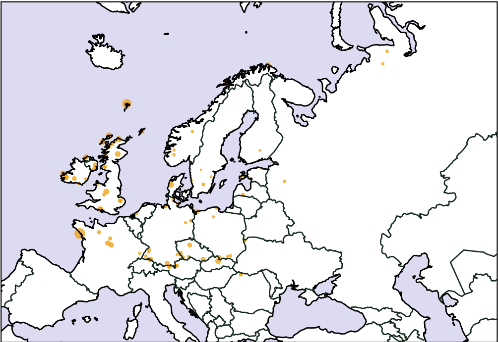
8000-6000 BP
