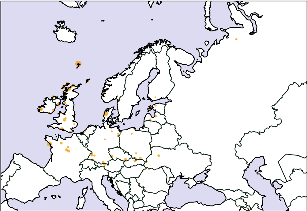
10000-8000 BP
