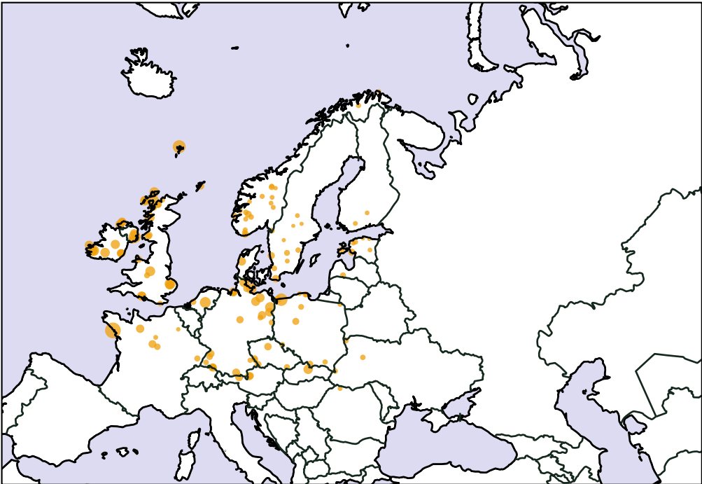
6000-4000 BP
