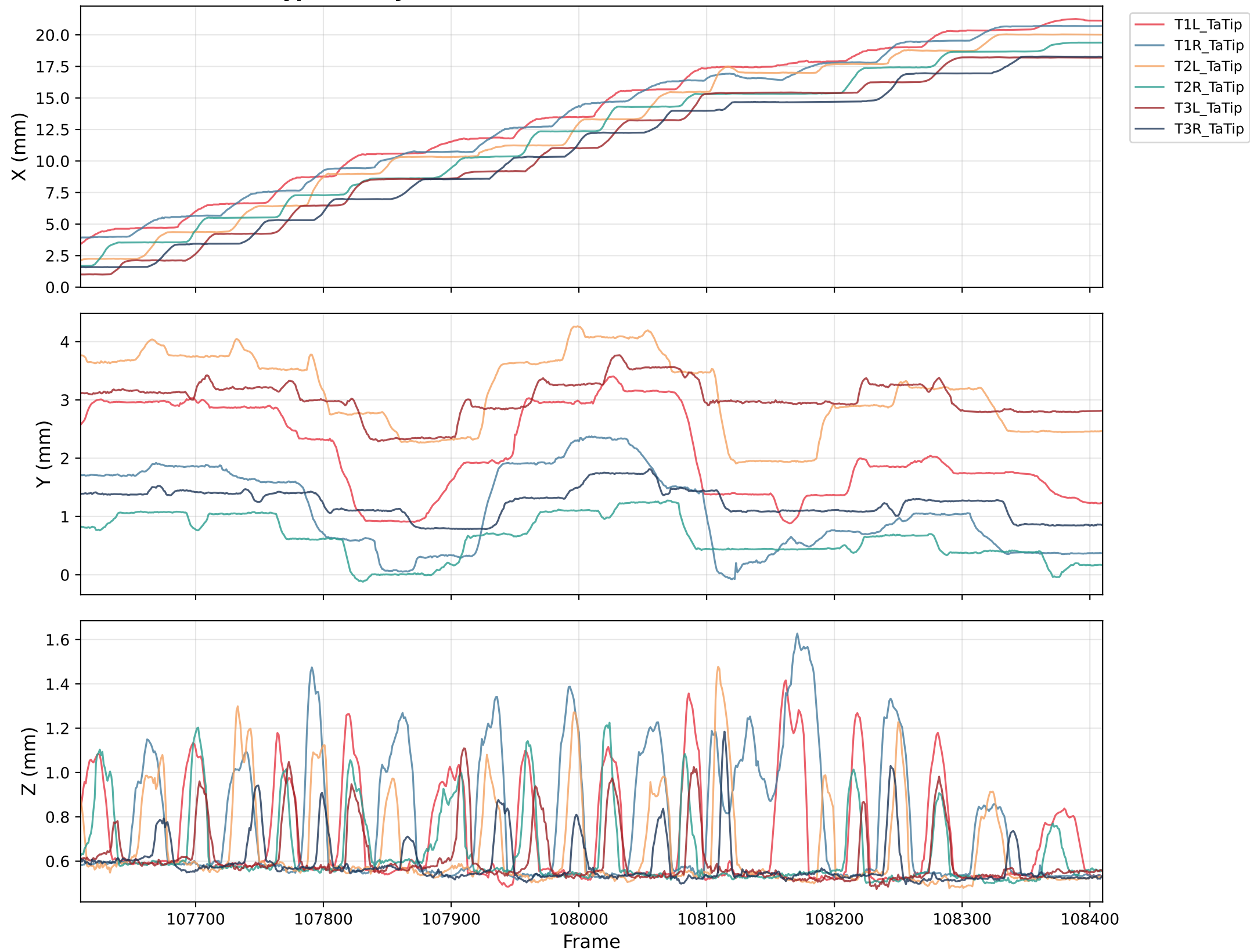
Keypoint Trajectories - Actual mm (Frames 107610-108410)
