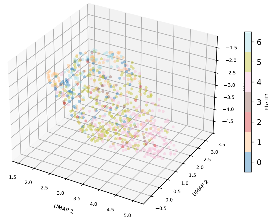
Fly ID
