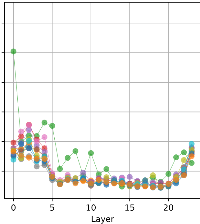
BLOOM-560M
