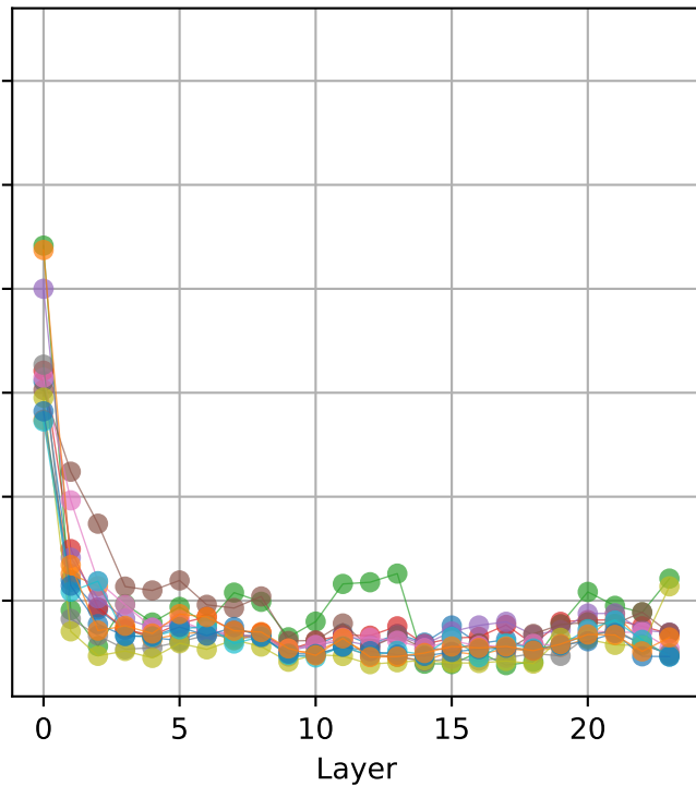
OPT-350M
