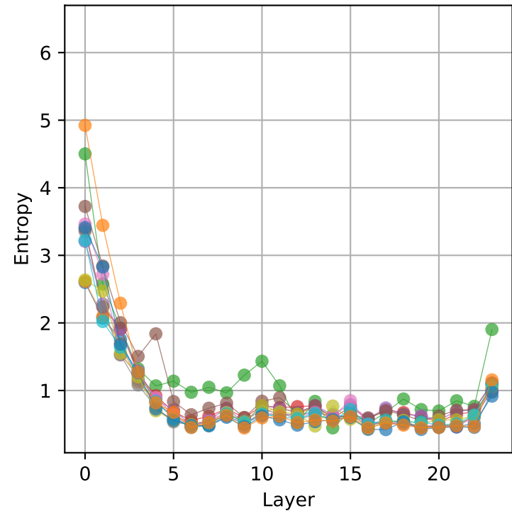
GPT-2 Medium
