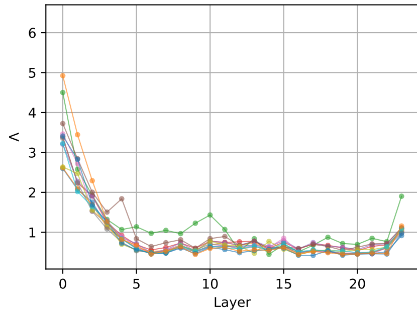
OPT-350M
