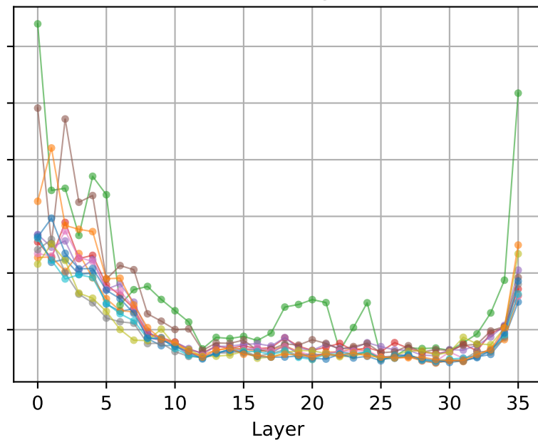
BLOOM-560M
