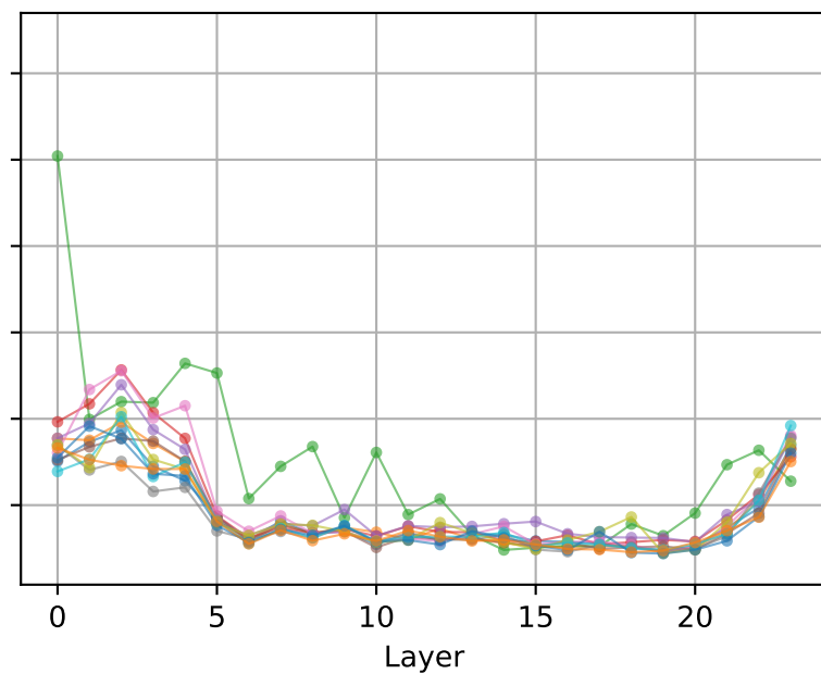
BLOOM-560M
