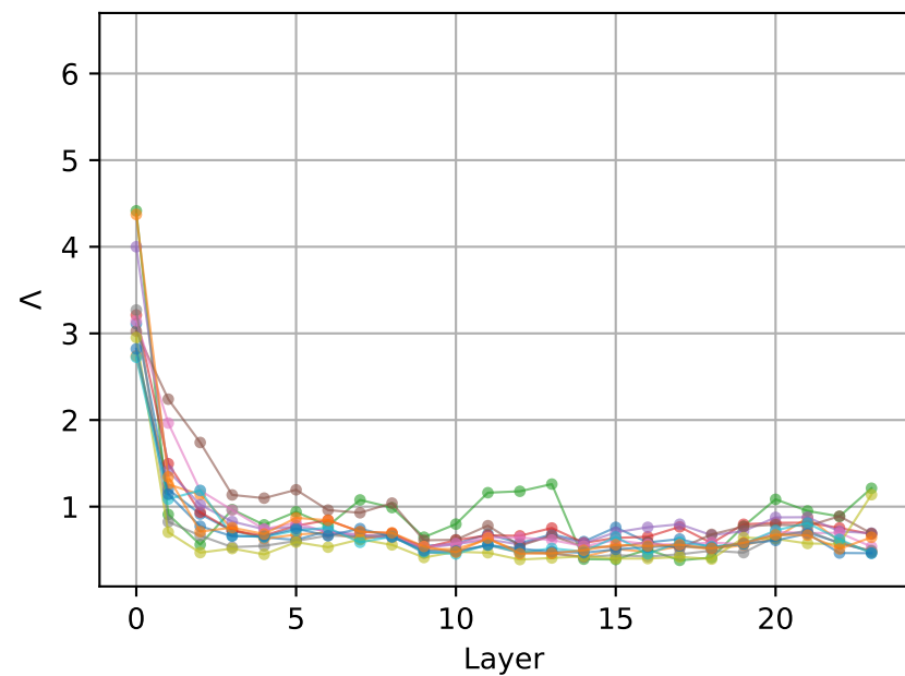
OPT-350M
