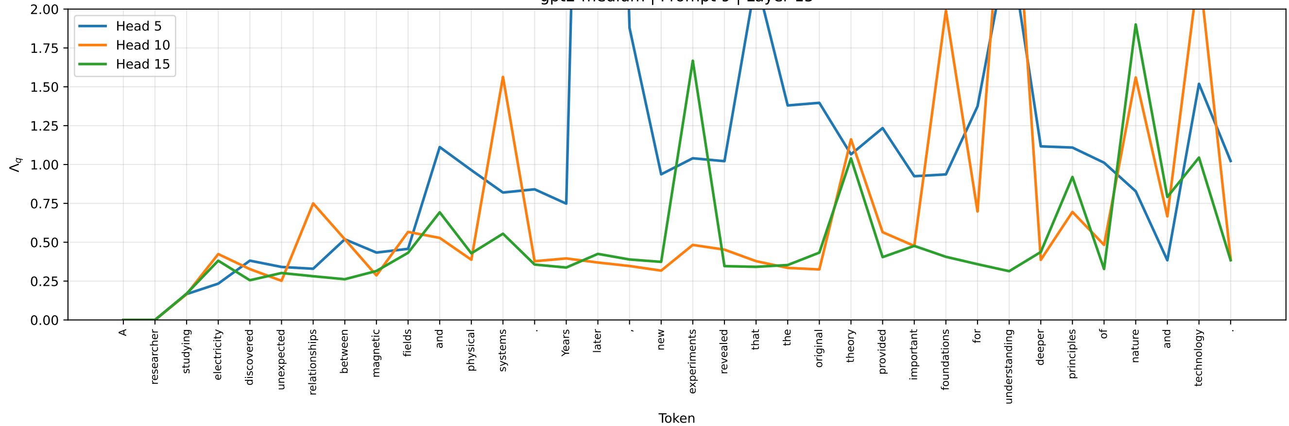
gpt2-medium | Prompt 9 | Layer 15
