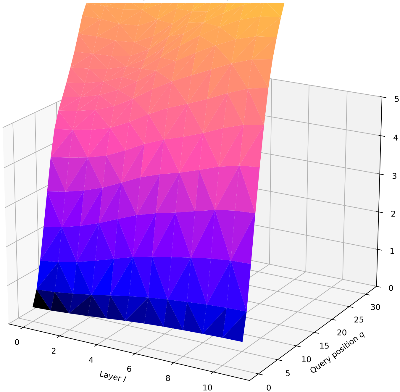
Pythia-410M — step16
