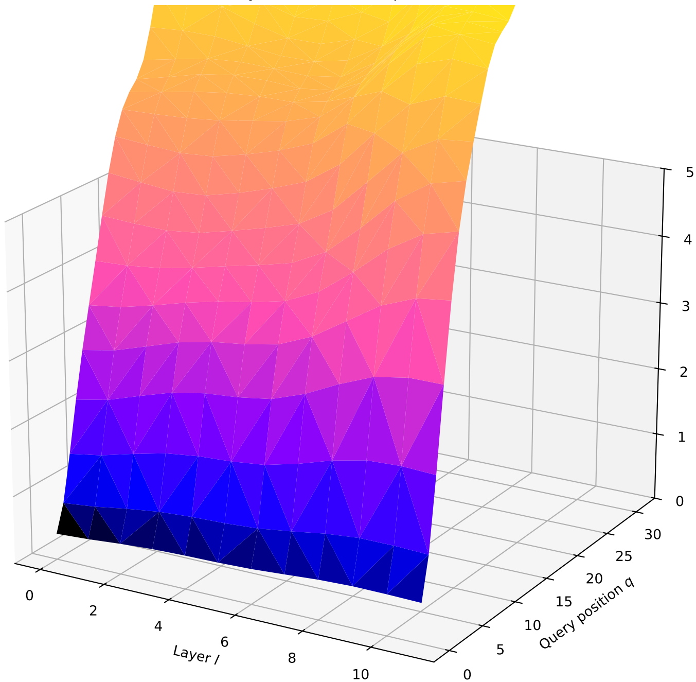
Pythia-410M — step64
