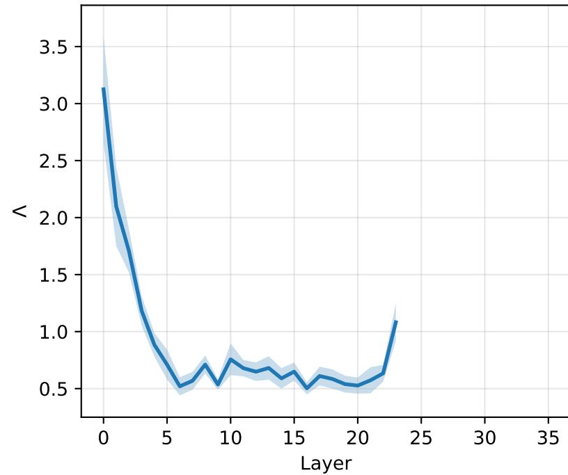
GPT-2 Medium
