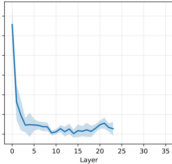
OPT-350M
