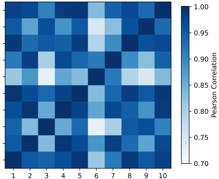
OPT-350M
