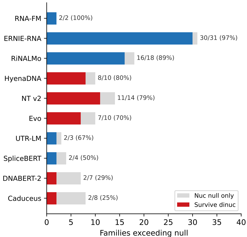
A. Dinucleotide null retention
