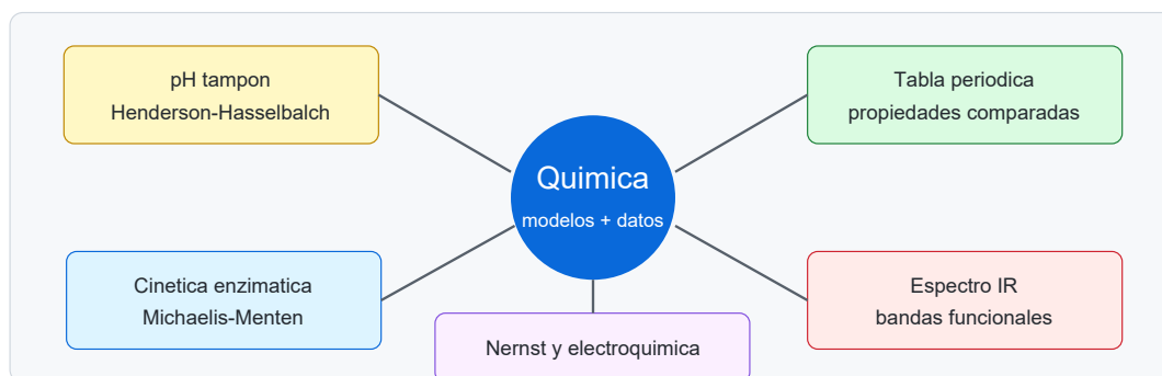
Figura12.1: Mapa de recursos docentes de la sección de Química.
