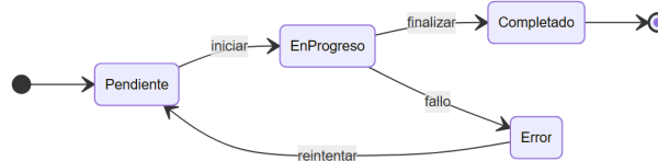
Figura26.5: Diagrama: Diagrama de estados (stateDiagram-v2).
