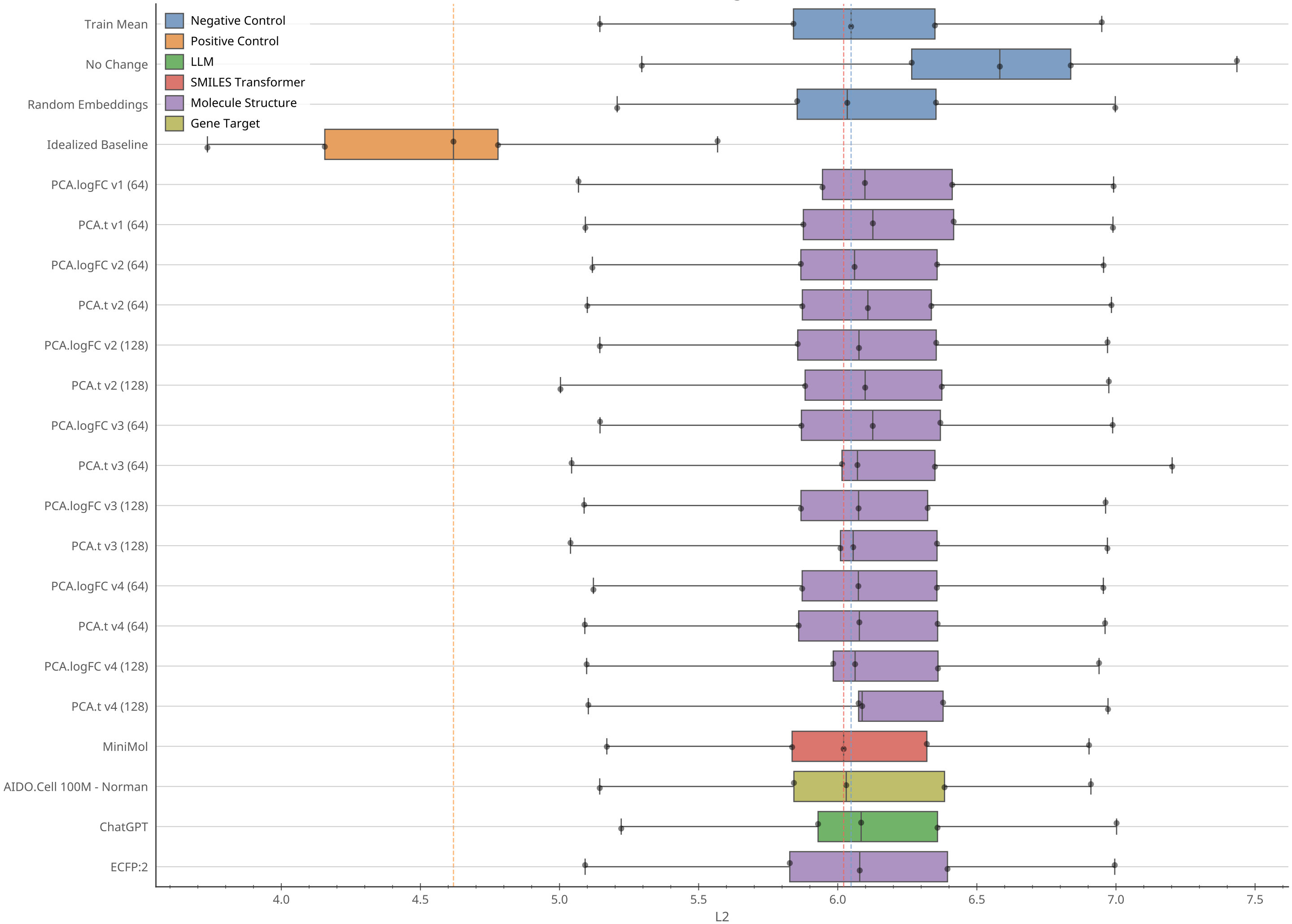
Tahoe LFC - KNN (PCA Embeddings, Dose 3.33 uM, CVCL_0320)
