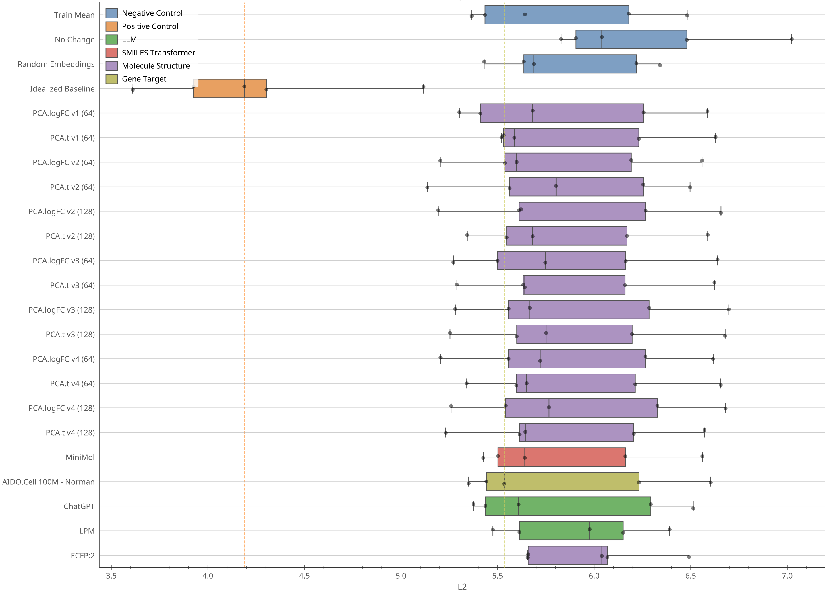
Tahoe LFC - KNN (PCA Embeddings + LPM, Dose 10 uM, CVCL_0023)
