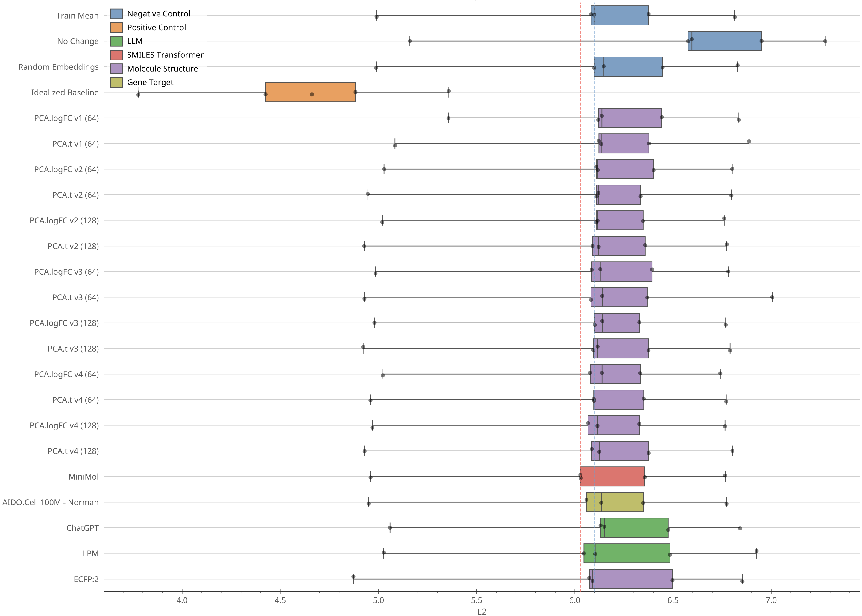
Tahoe LFC - KNN (PCA Embeddings + LPM, Dose 3.33 uM, CVCL_0320)
