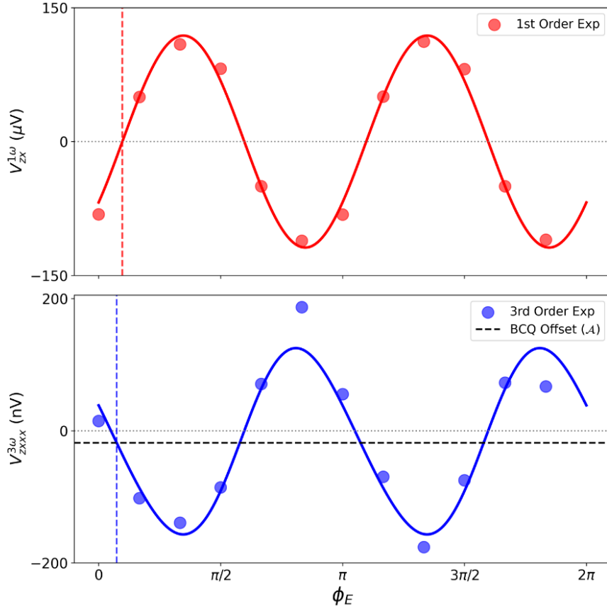
图 4.1 一阶（ 1\omega ）与三阶（ 3\omega ）Hall 电压的联合角度拟合。红蓝虚线分别标示各自相对于拟合偏移的零交叉点。三阶谐波相对于一阶的微小相位偏移来源于
