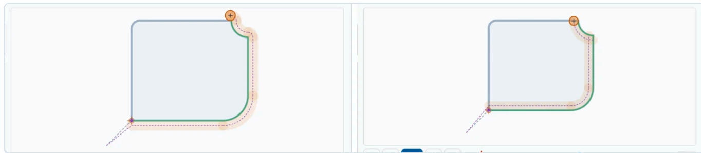
Figura 50. La simulación con compensación: con G42 (izquierda) el camino del centro de la fresa —morado— y su huella van por fuera de la pieza; con G41 (derecha), por dentro: se la come.
