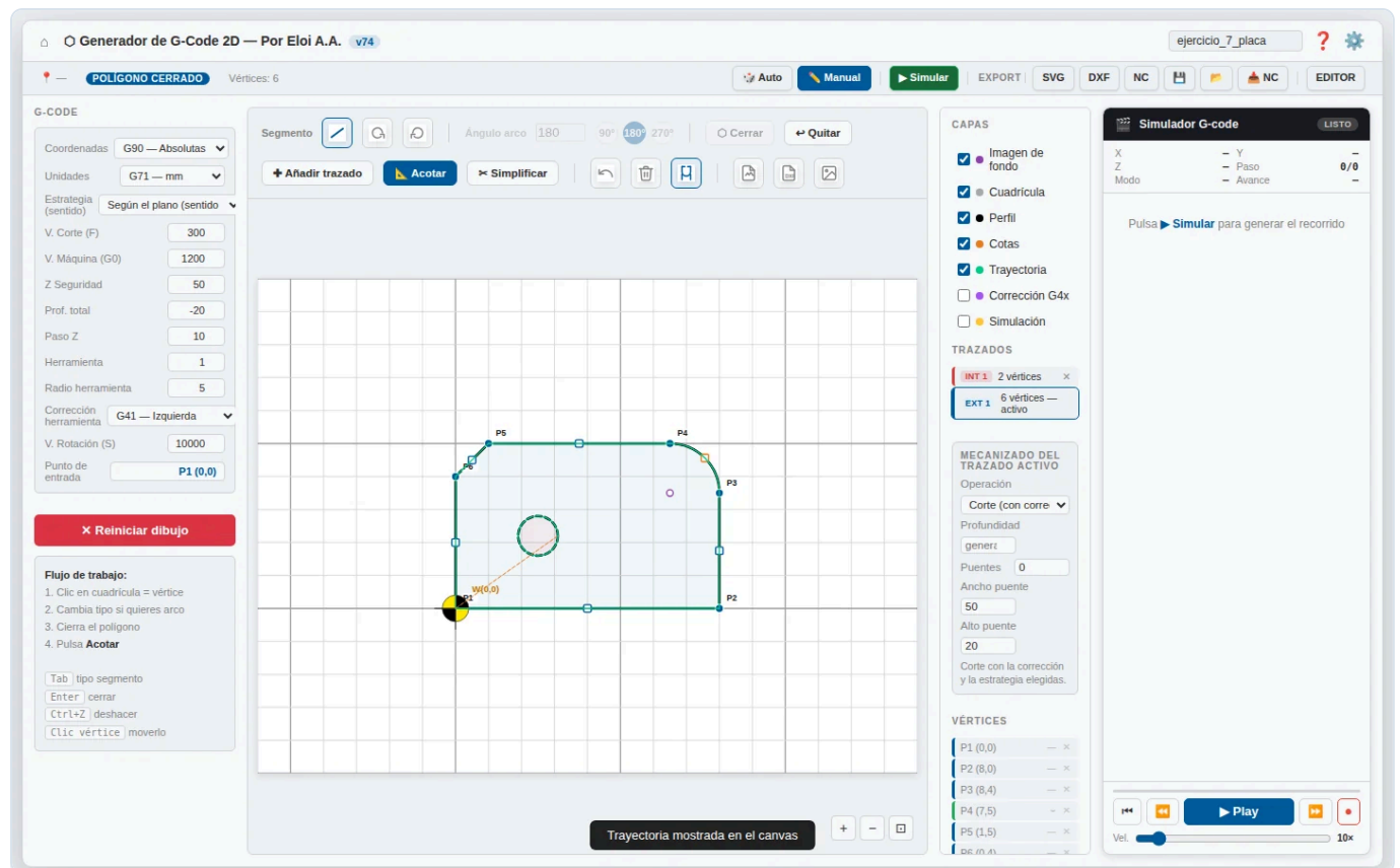
Figura 54. La placa del tutorial abierta en el Generador, con su cero pieza W en el mismo sitio que en el plano.
