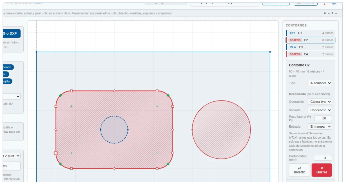
Figura 51. Una placa con dos cajeras (rayadas): la de la izquierda, concéntrica y con una isla (en blanco, con línea discontinua); la de la derecha, en zigzag.
