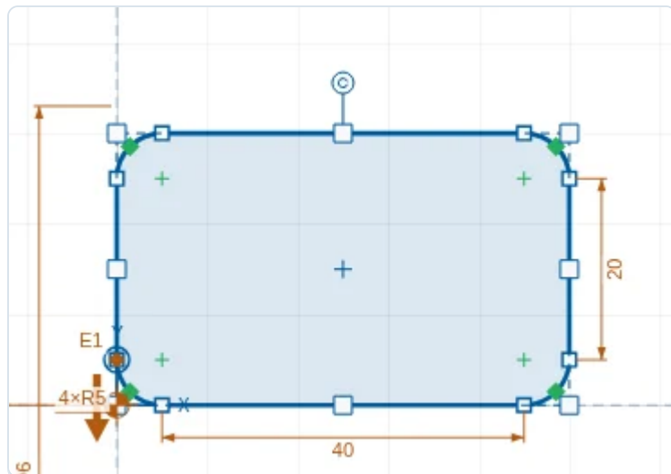
Figura 29. Marco de transformación: asas de esquina y de lado, asa de giro arriba y centro.
