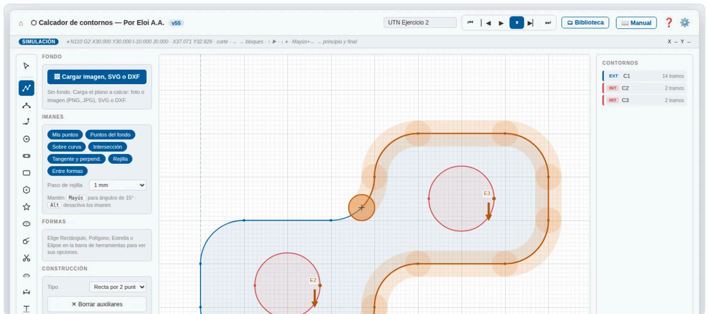
Figura 51. El reproductor de la barra superior: la fresa recorre el contorno exterior, con su huella; en la barra de estado, el bloque en curso.
