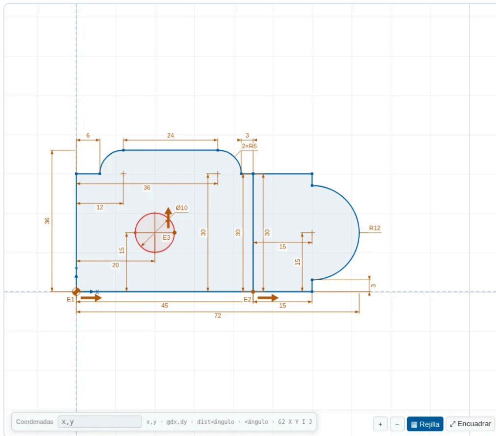
Figura 31. Después: fusionados, con un taladro restado y partidos con una línea en dos piezas.
