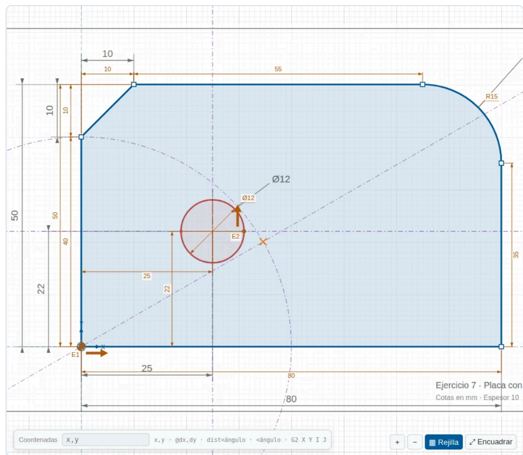
Figura 24. Una recta a 30° y un círculo de R40 desde el cero pieza; el imán marca su intersección (X).
