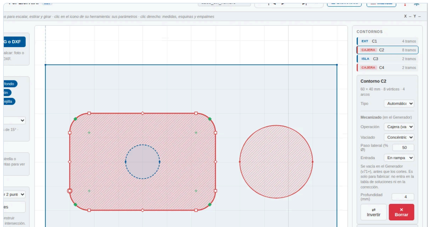
Figura 50. Una placa con dos cajeras (rayadas): la de la izquierda, concéntrica y con una isla (en blanco, con línea discontinua); la de la derecha, en zigzag.
