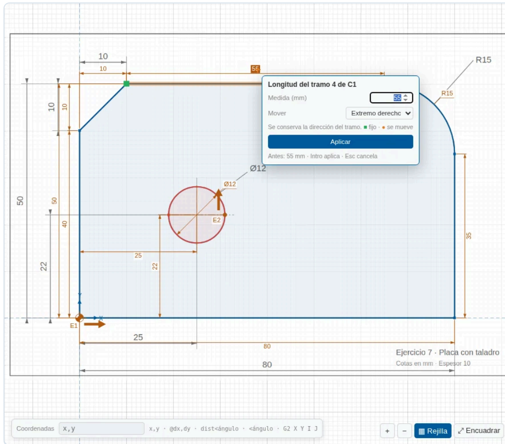
Figura 6. Doble clic en una cota: se escribe la medida del plano y se elige qué extremo se mueve.
