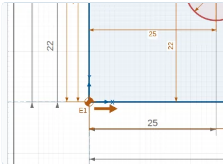
Figura 7. Cero pieza, punto de entrada E1 y flecha de sentido.
