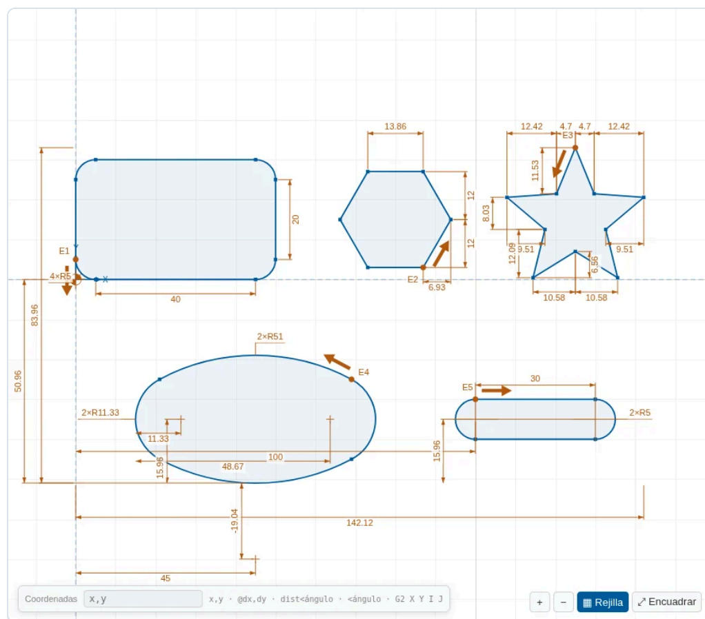
Figura 17. Rectángulo con esquinas redondeadas, hexágono de 24 entre caras, estrella, elipse (óvalo) y ranura, con sus cotas.
