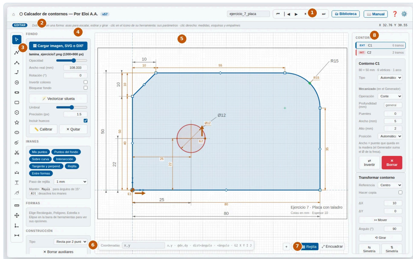
Figura 1. Las zonas de la pantalla del programa.
