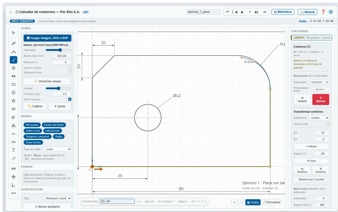
Figura 4. Dibujando el arco tangente; la caja de coordenadas muestra el punto que se va a añadir.
