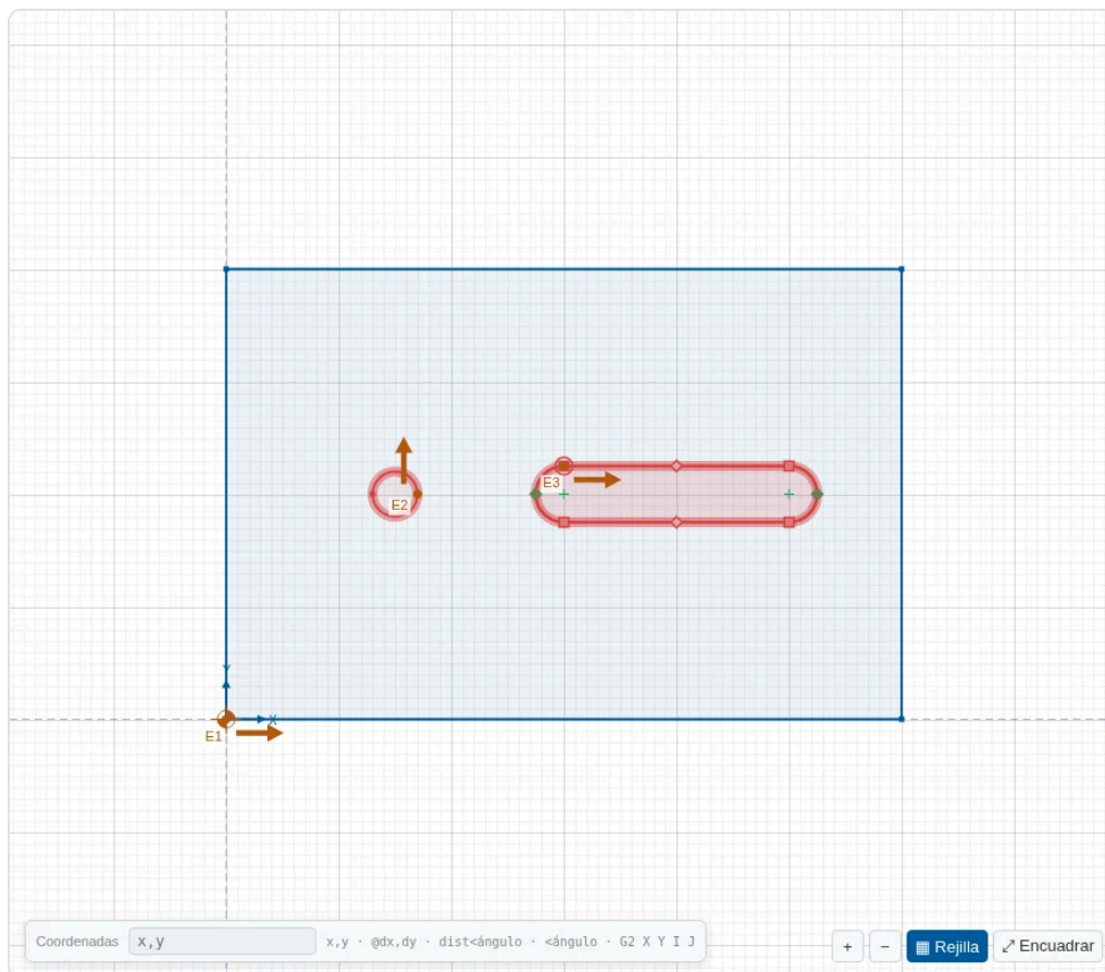
Figura 36. Con una fresa de \varnothing 6 , el taladro de \varnothing 4 y la ranura de 5 mm quedan en rojo.
