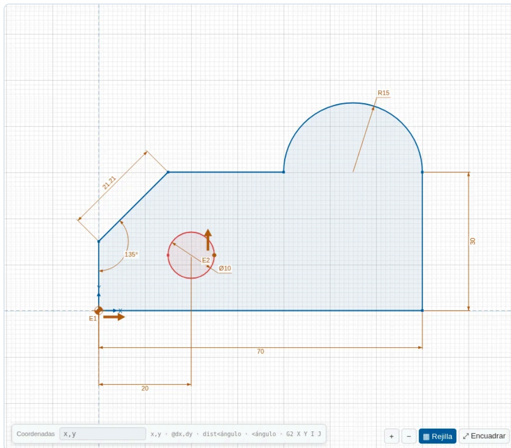
Figura 35. Un plano acotado solo con cotas manuales: horizontales, vertical, alineada, ángulo, radio, diámetro y posición del taladro.
