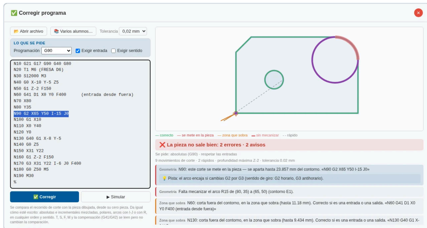
Figura 47. Corrección de un programa en el que el alumno ha escrito G2 en lugar de G3 en el bloque N90: el arco sale hacia dentro de la pieza, queda un tramo sin mecanizar y la pista indica la causa.
