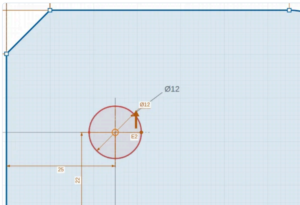
Figura 16. El imán de centro engancha exactamente el centro del taladro.
