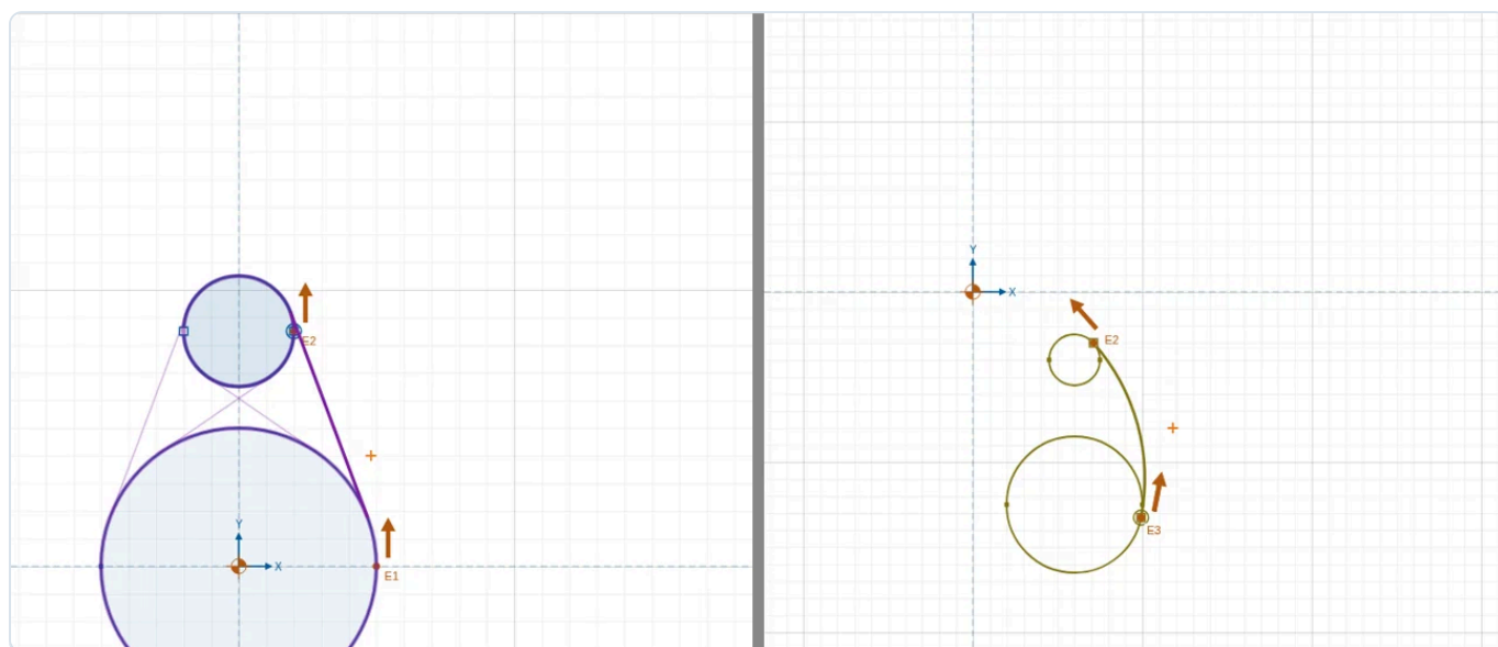
Figura 25. A la izquierda, las cuatro rectas tangentes a dos círculos (la resaltada es la que se creará); a la derecha, un arco R120 tangente a dos círculos, que han quedado cortados en las tangencias.
