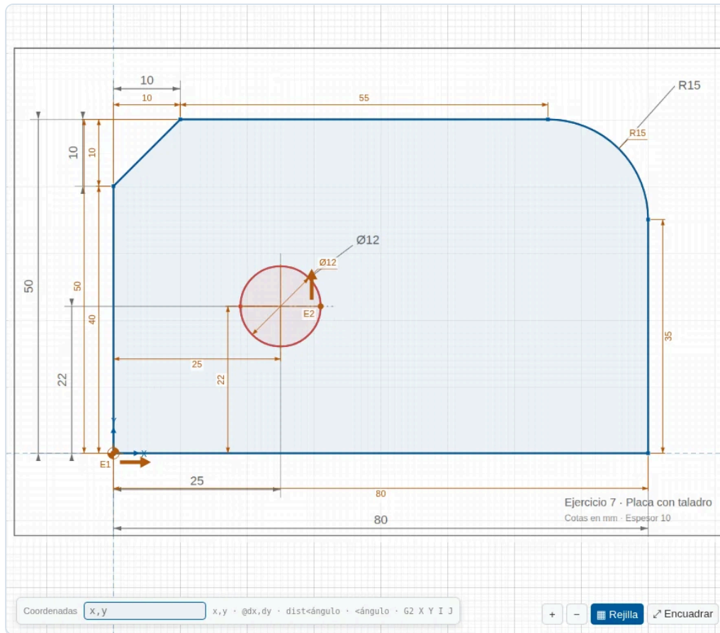
Figura 5. La pieza calcada con sus cotas automáticas sobre la lámina.
