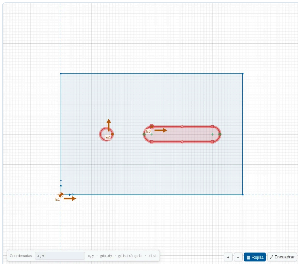
Figura 34. Con una fresa de Ø6, el taladro de Ø4 y la ranura de 5 mm quedan en rojo.
