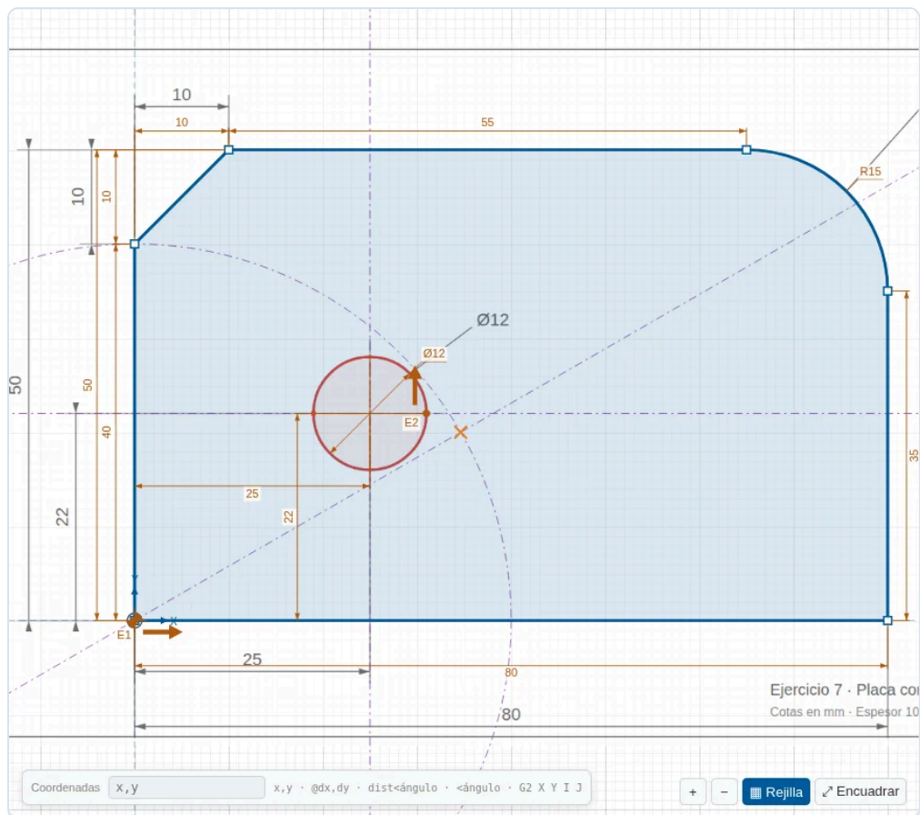
Figura 24. Una recta a 30° y un círculo de R40 desde el cero pieza; el imán marca su intersección (X).
