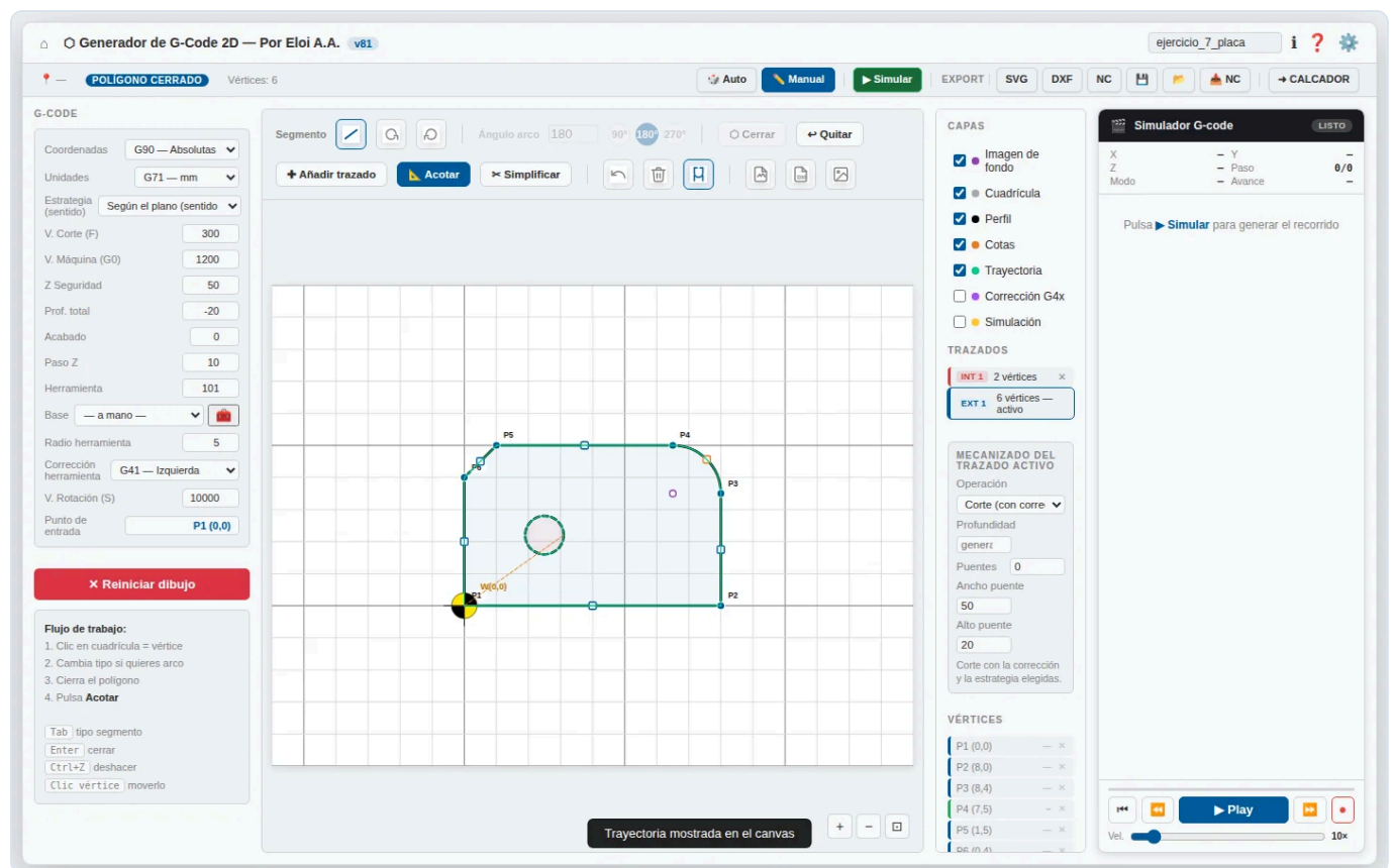
Figura 54. La placa del tutorial abierta en el Generador, con su cero pieza W en el mismo sitio que en el plano.
