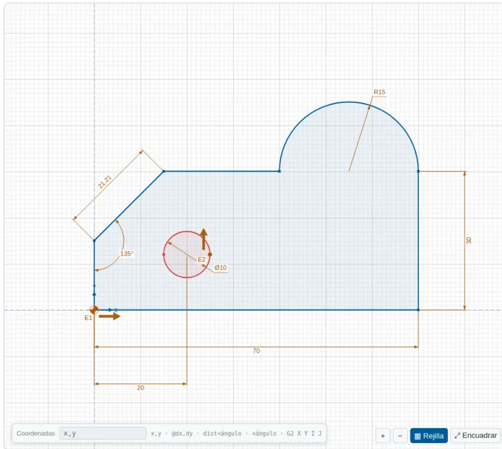
Figura 35. Un plano acotado solo con cotas manuales: horizontales, vertical, alineada, ángulo, radio, diámetro y posición del taladro.
