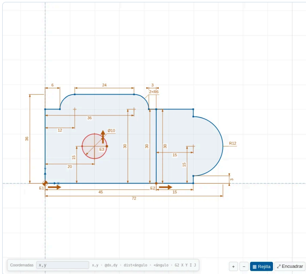
Figura 31. Después: fusionados, con un taladro restado y partidos con una línea en dos piezas.
