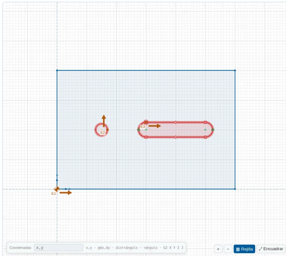
Figura 36. Con una fresa de \varnothing 6 , el taladro de \varnothing 4 y la ranura de 5 mm quedan en rojo.
