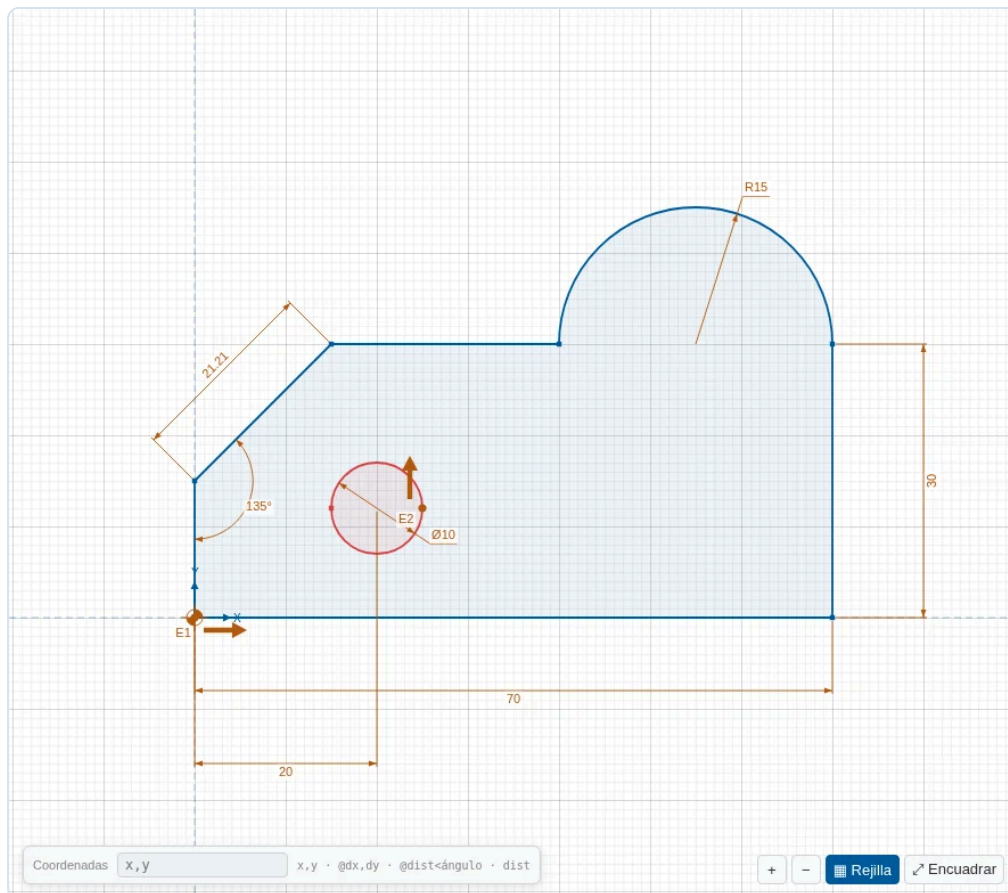
Figura 33. Un plano acotado solo con cotas manuales: horizontales, vertical, alineada, ángulo, radio, diámetro y posición del taladro.
