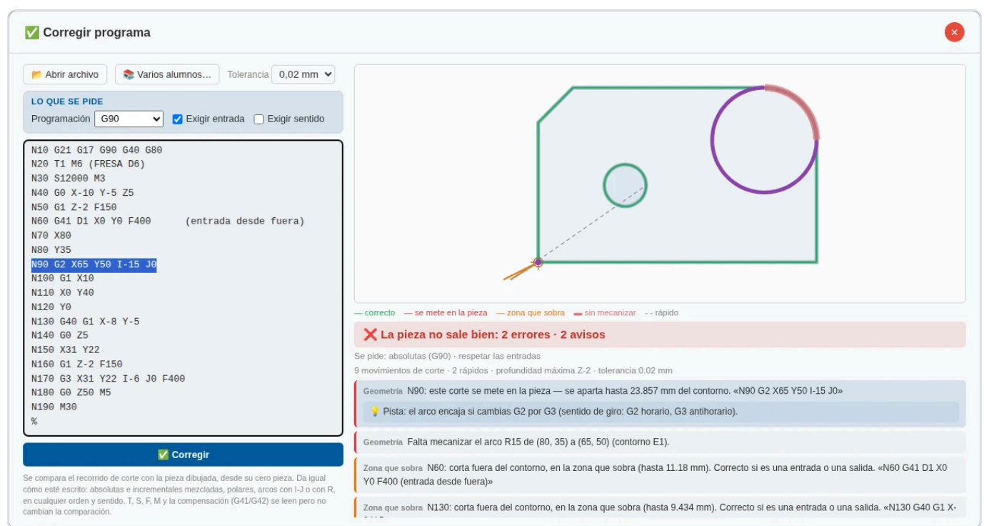
Figura 42. Corrección de un programa en el que el alumno ha escrito G2 en lugar de G3 en el bloque N90: el arco sale hacia dentro de la pieza, queda un tramo sin mecanizar y la pista indica la causa.
