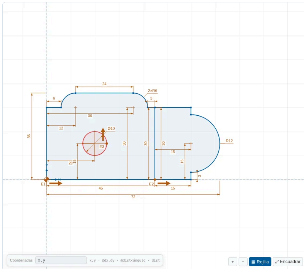
Figura 29. Después: fusionados, con un taladro restado y partidos con una línea en dos piezas.
