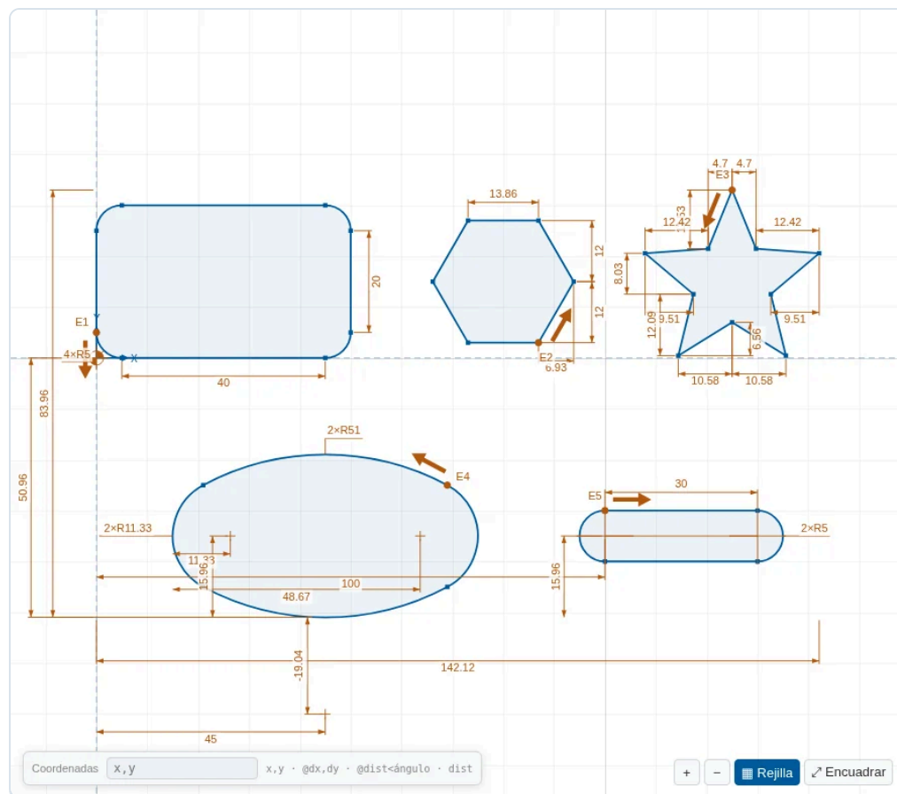
Figura 17. Rectángulo con esquinas redondeadas, hexágono de 24 entre caras, estrella, elipse (óvalo) y ranura, con sus cotas.
