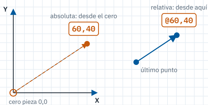
Figura 8. Sin arroba, el punto se mide desde el cero pieza; con arroba, desde el último punto marcado.
