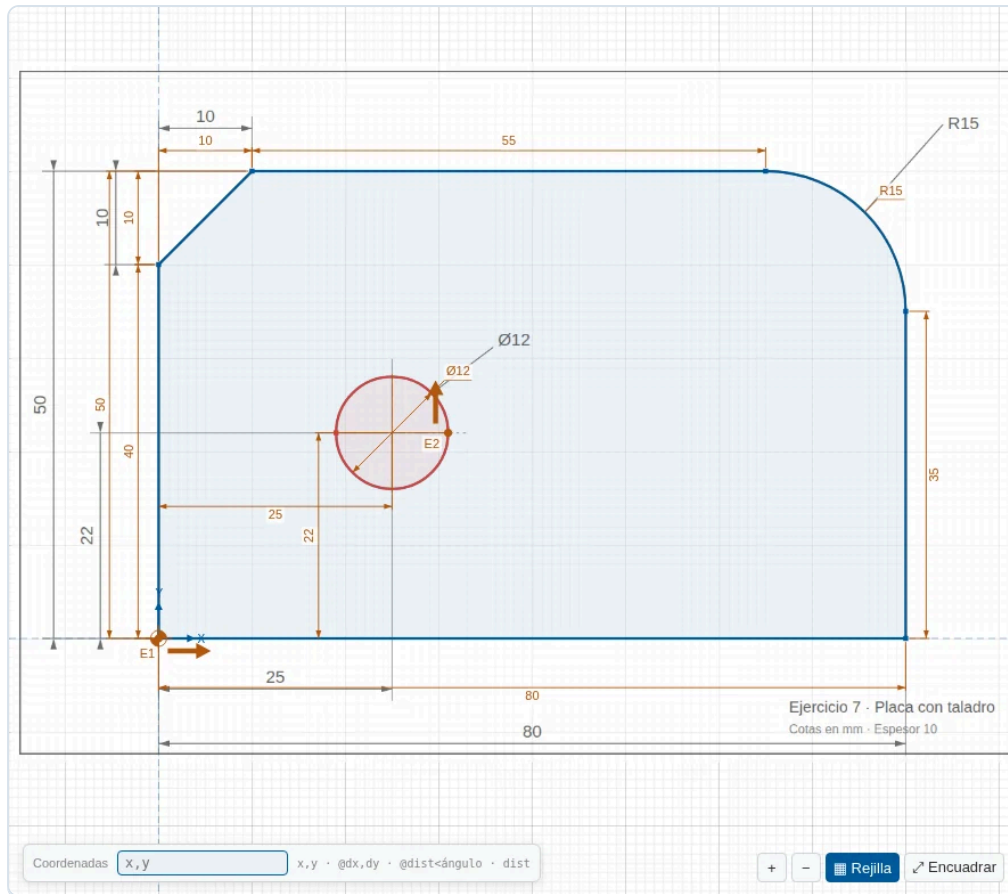
Figura 5. La pieza calcada con sus cotas automáticas sobre la lámina.
