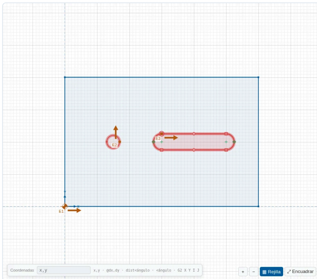
Figura 36. Con una fresa de Ø6, el taladro de Ø4 y la ranura de 5 mm quedan en rojo.
