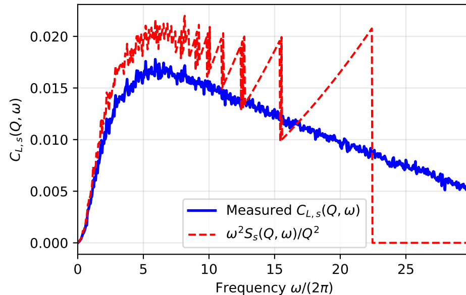
Self Longitudinal C_{L,s}(Q, \omega) ( Q = 0.977 )
