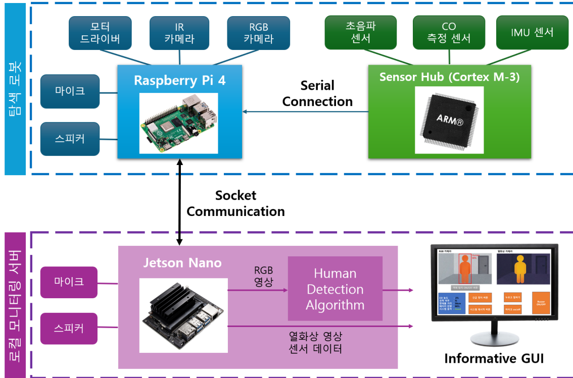
그림 2. 탐색 로봇 / 모니터링 컴퓨터 구성도
