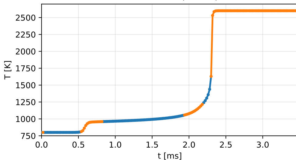
lambda_init=1.0 CVODE 49% (n=175)
