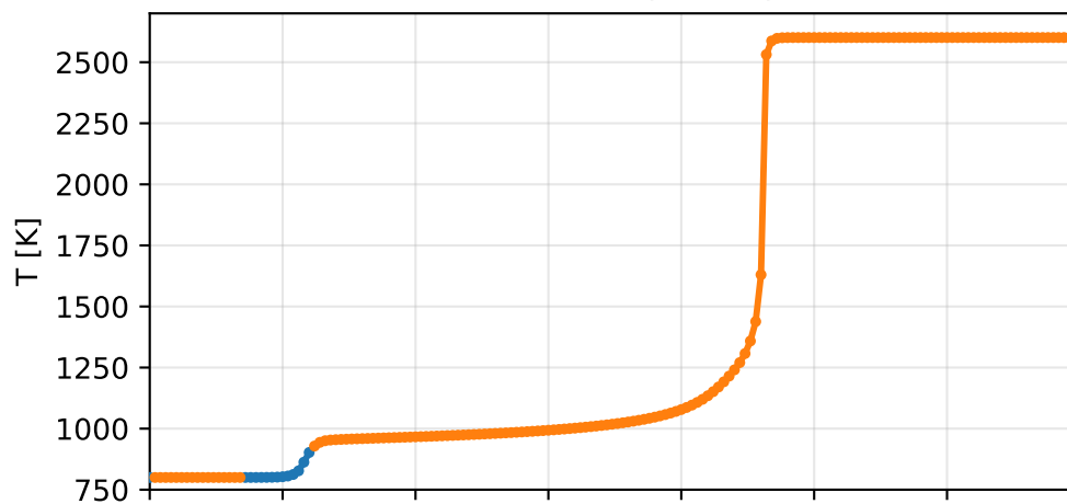
lambda_init=1.0 CVODE 49% (n=175)
