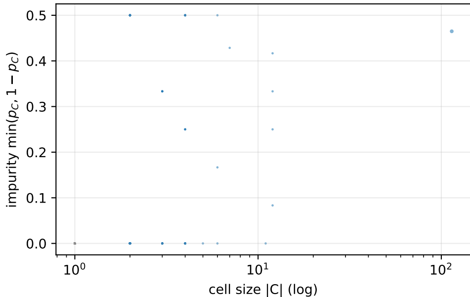
E3 cell scatter: cora, L=2 (K=2301, singletons=2127)
