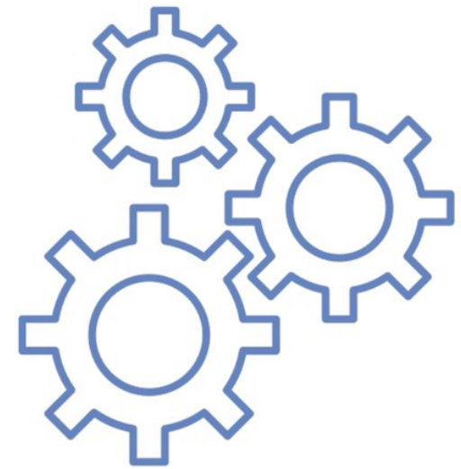
Moteur JavaScript
