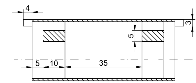
A-A
