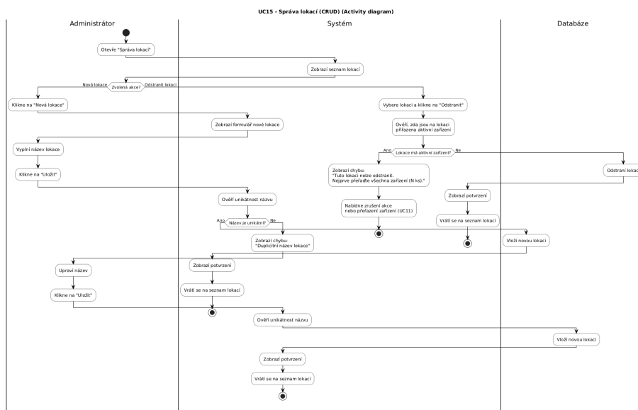
Obrázek 4: Activity diagram pro UC15 – Správa lokací (CRUD)
