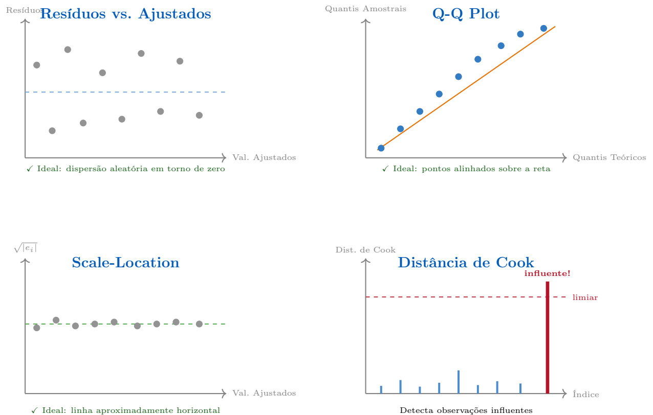
Figura 4: Quatro gráficos diagnósticos padrão para regressão. Superior esq.: resíduos sem padrão indicam bom ajuste. Superior dir.: normalidade dos resíduos pelo Q-Q plot. Inferior esq.: homocedasticidade (variância constante). Inferior dir.: Cook's Distance identifica pontos influentes.
