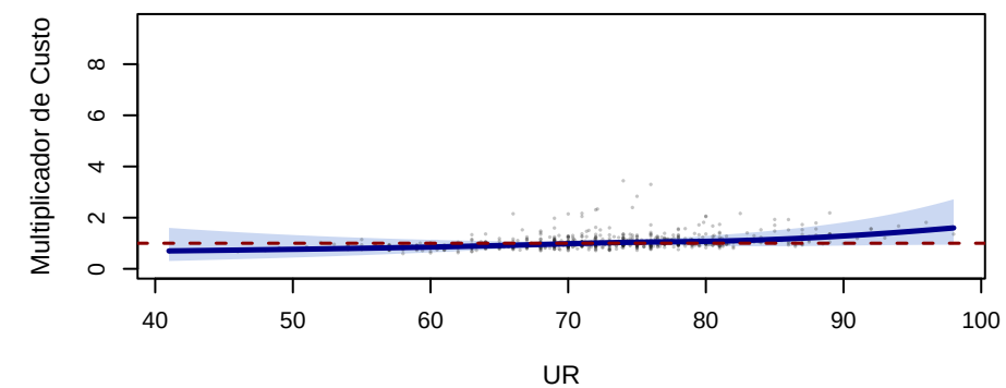
s(UR,3.66)
