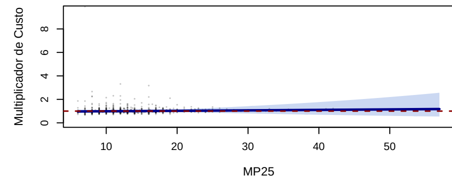
s(MP25,0.99)
