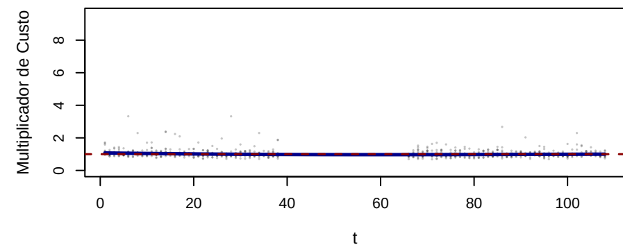
s(t,2.41)
