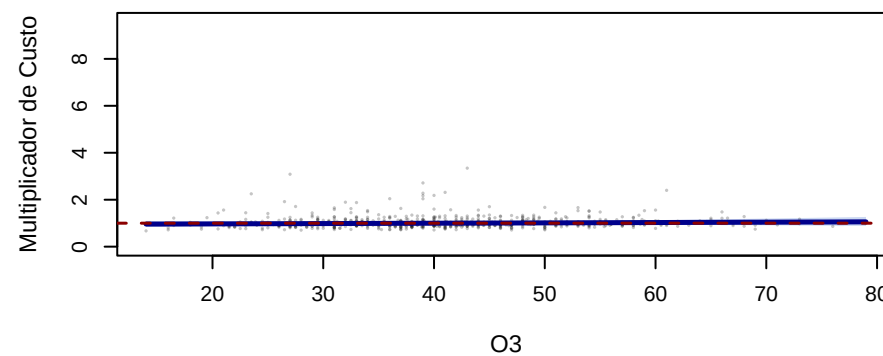
s(O3,1.04)
