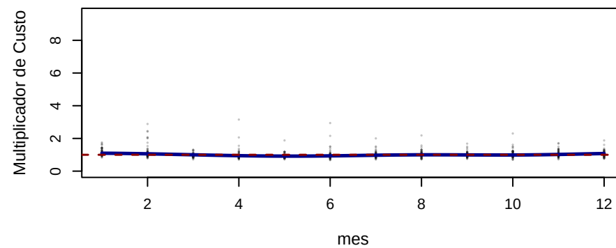
s(mes,3.65)
