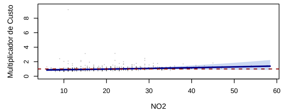
s(NO2,1.05)
