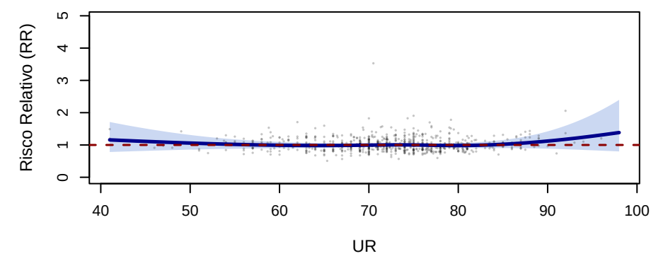
s(UR,3.74)
