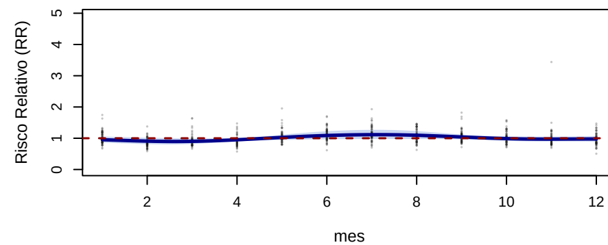
s(mes,3.77)
