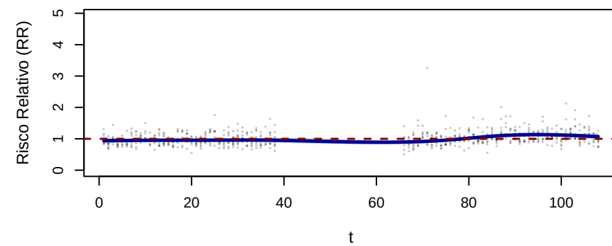
s(t,5.68)
