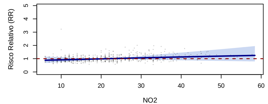
s(NO2,1.72)
