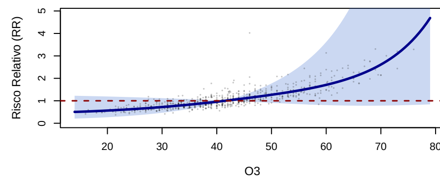
s(O3,3)
