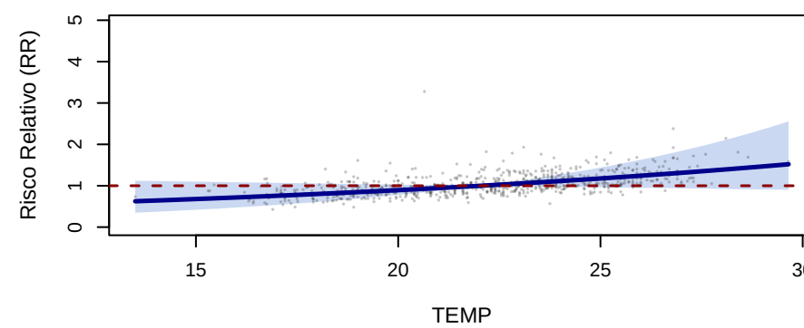
s(TEMP,1)
