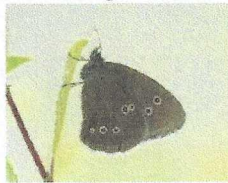
Ringlet
