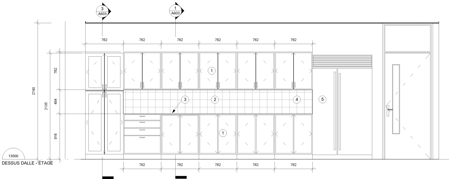
ÉLEVATION-COMPTOIR CUISINE
