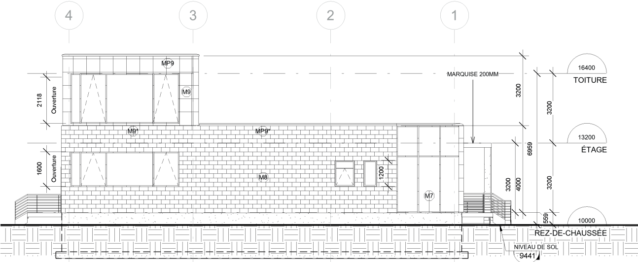
ÉLEVATION NORD
