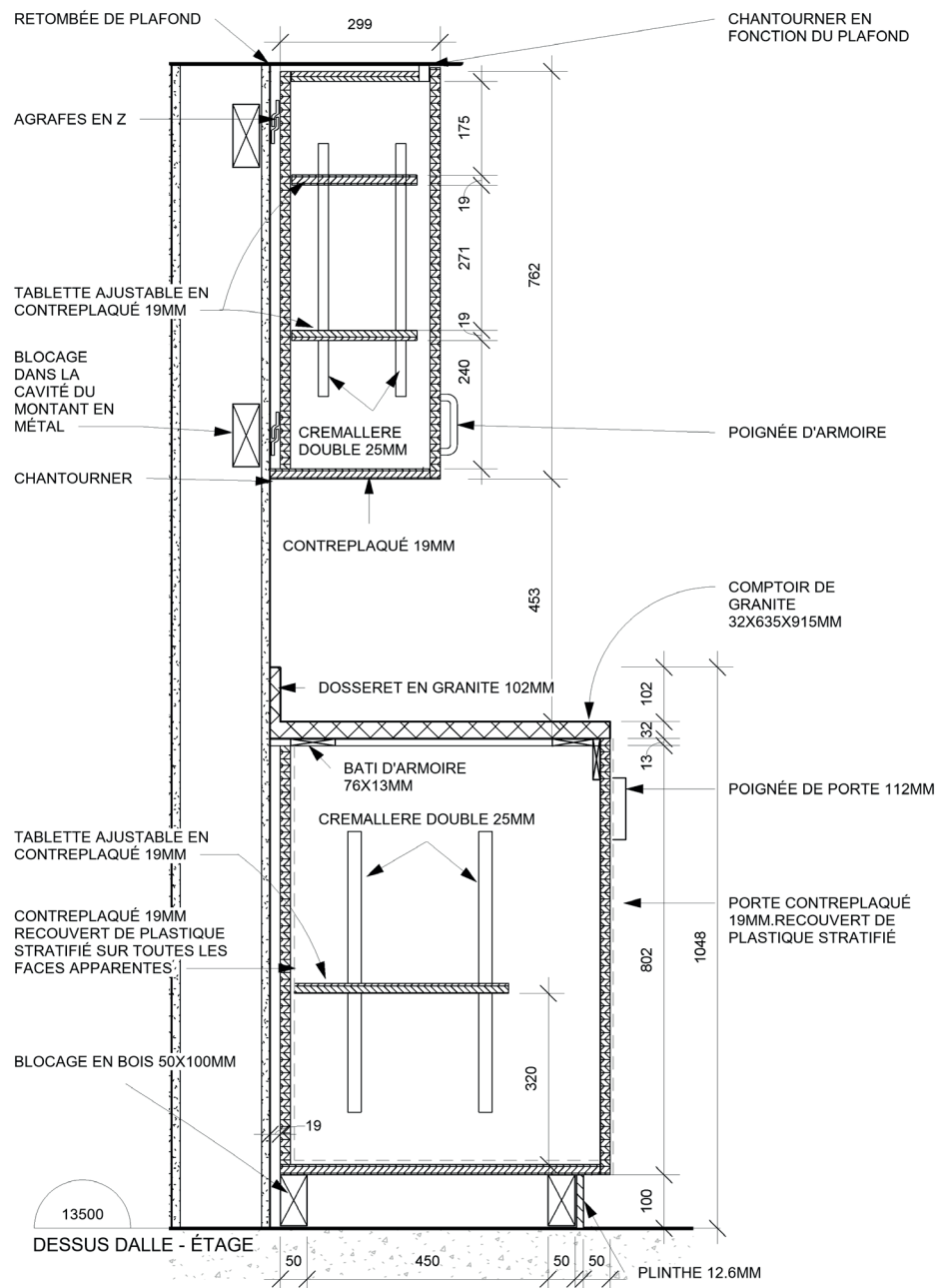
DÉTAILS ARMOIRES-BASSES ET ARMOIRES-HAUTES
