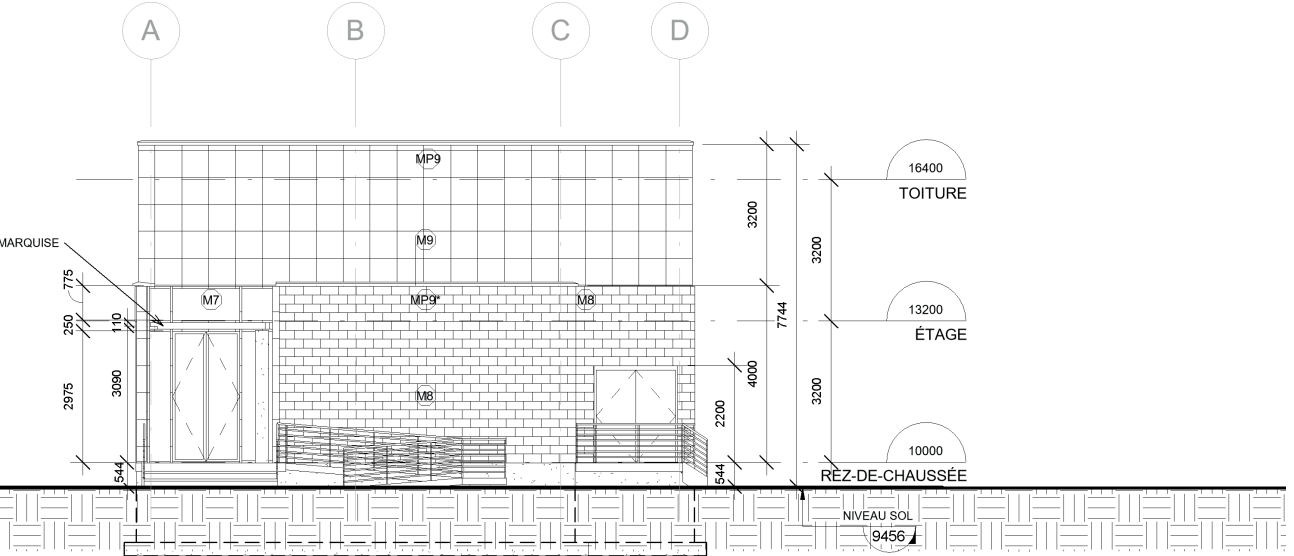
ÉLEVATION OUEST
