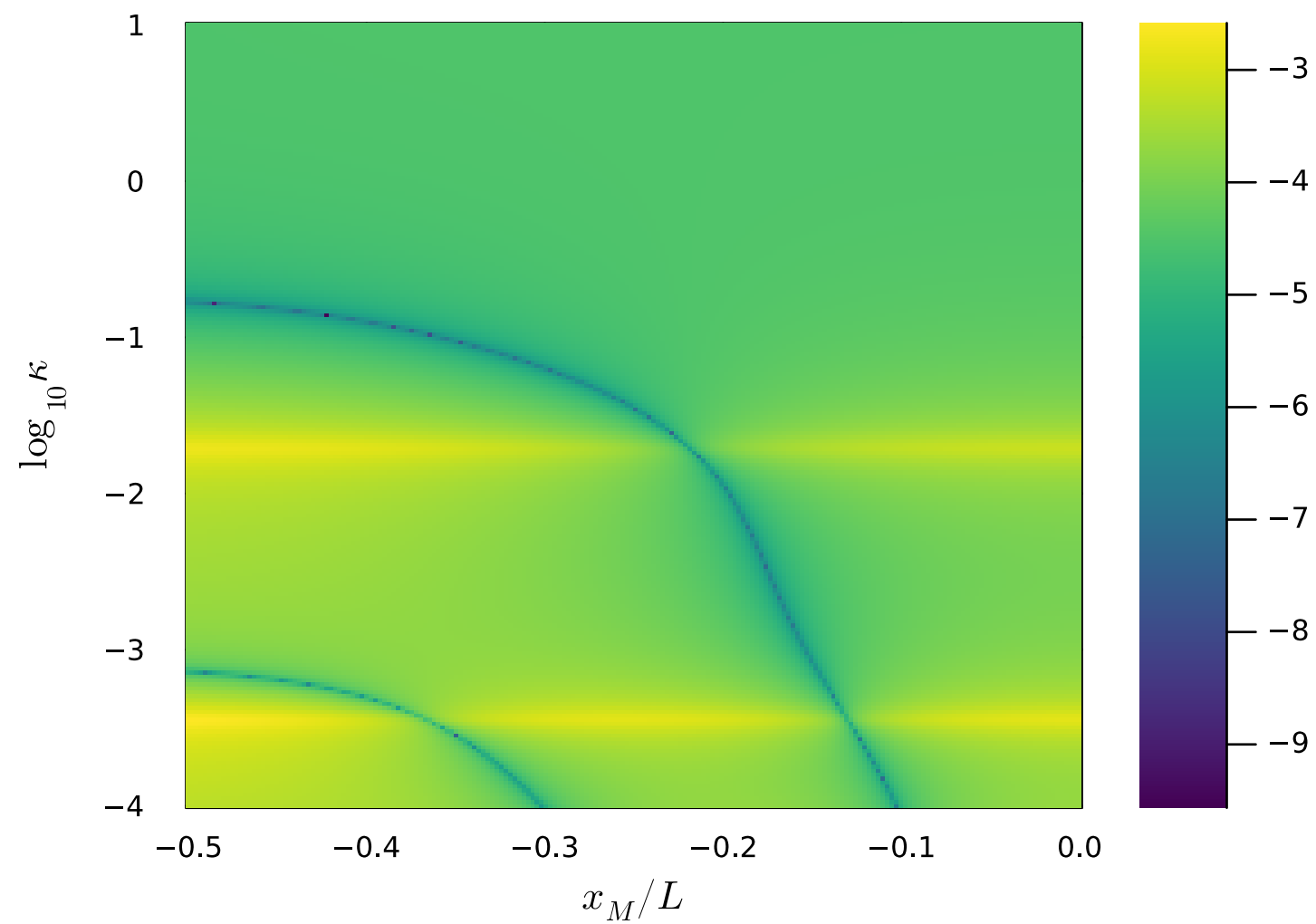
\log_{10}|S|
