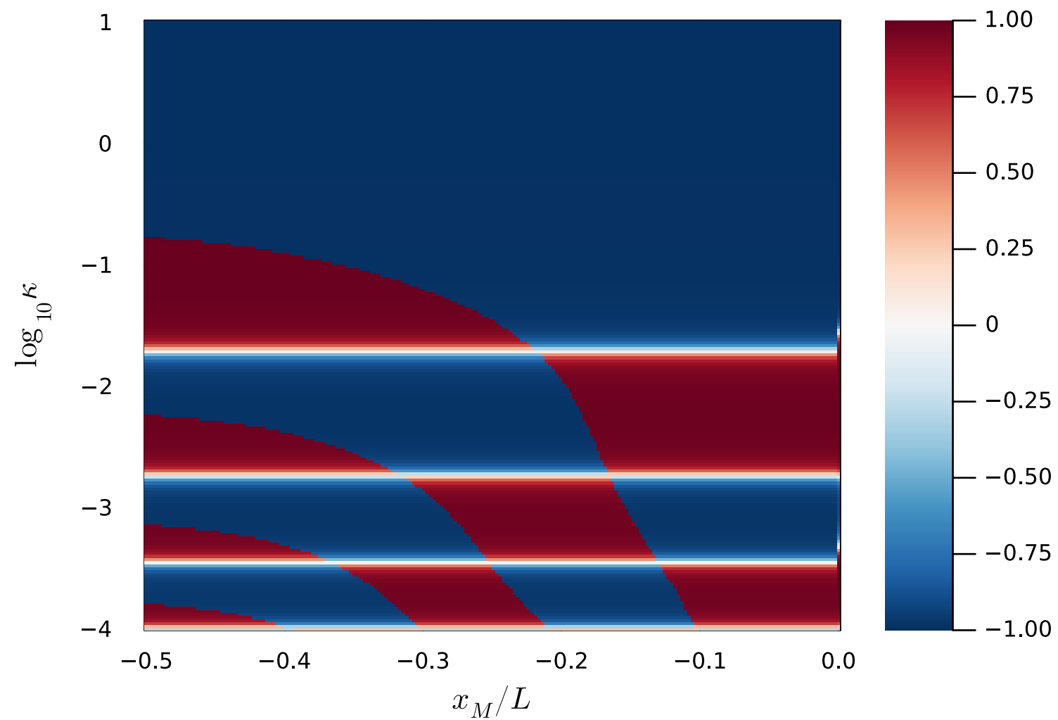
\cos(\arg S - \arg A)
