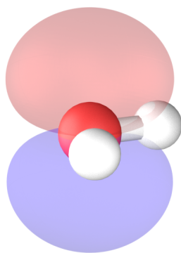
Figure 11.1: Orbital HOMO da água calculado usando o PySCF e visualizado no Blender
