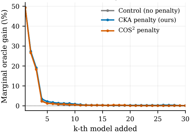
MMLU
