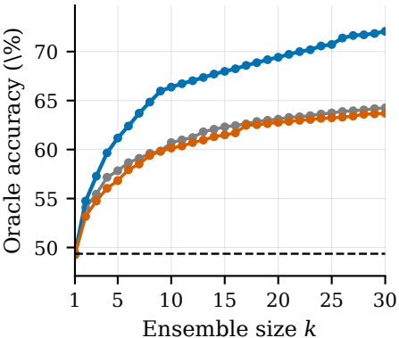
MMLU
