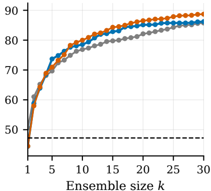
GSM8K
