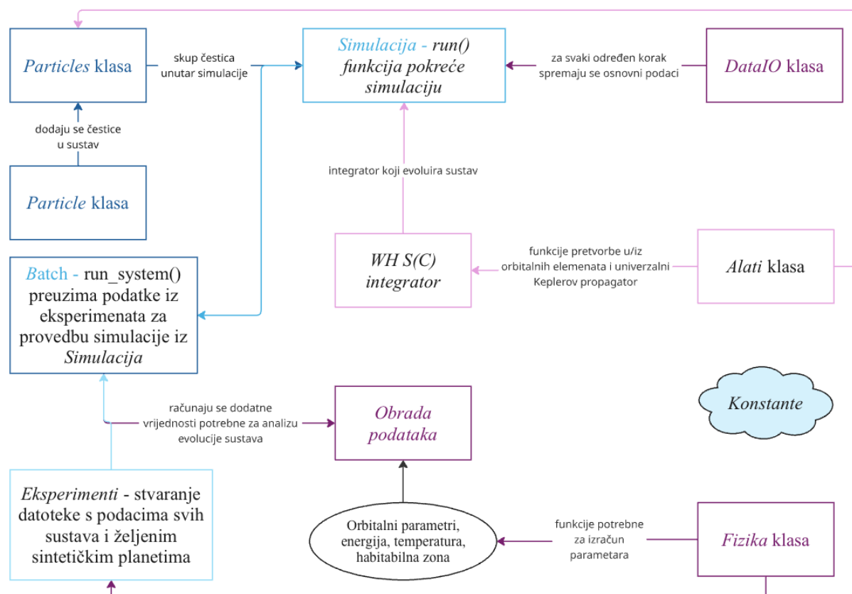
Slika 5: Grafički prikaz funkcionalnosti programa potrebnog za provedbu ovog rada, uključujući pomoćne klase za određivanje i spremanje čestica, spremanje podataka, potrebnih alata i funkcija za izračune, sam integrator te generacija eksperimenata za simulaciju. Određeni dijelovi programa po uzoru na [4]. Ilustracija autora.
