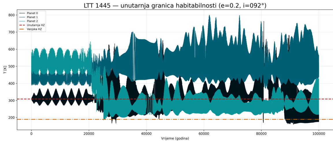
Slika 18: ovisnost temperature o vremenu za planete sustava LTT 1445. Crvena iscrtkana linija označava unutarnju granicu habitabilne zone, a žuta iscrtkana linija vanjsku granicu zone. Ovdje drugi planet postane habitabilniji tijekom evolucije, no raspon temperatura je izrazito velik.
