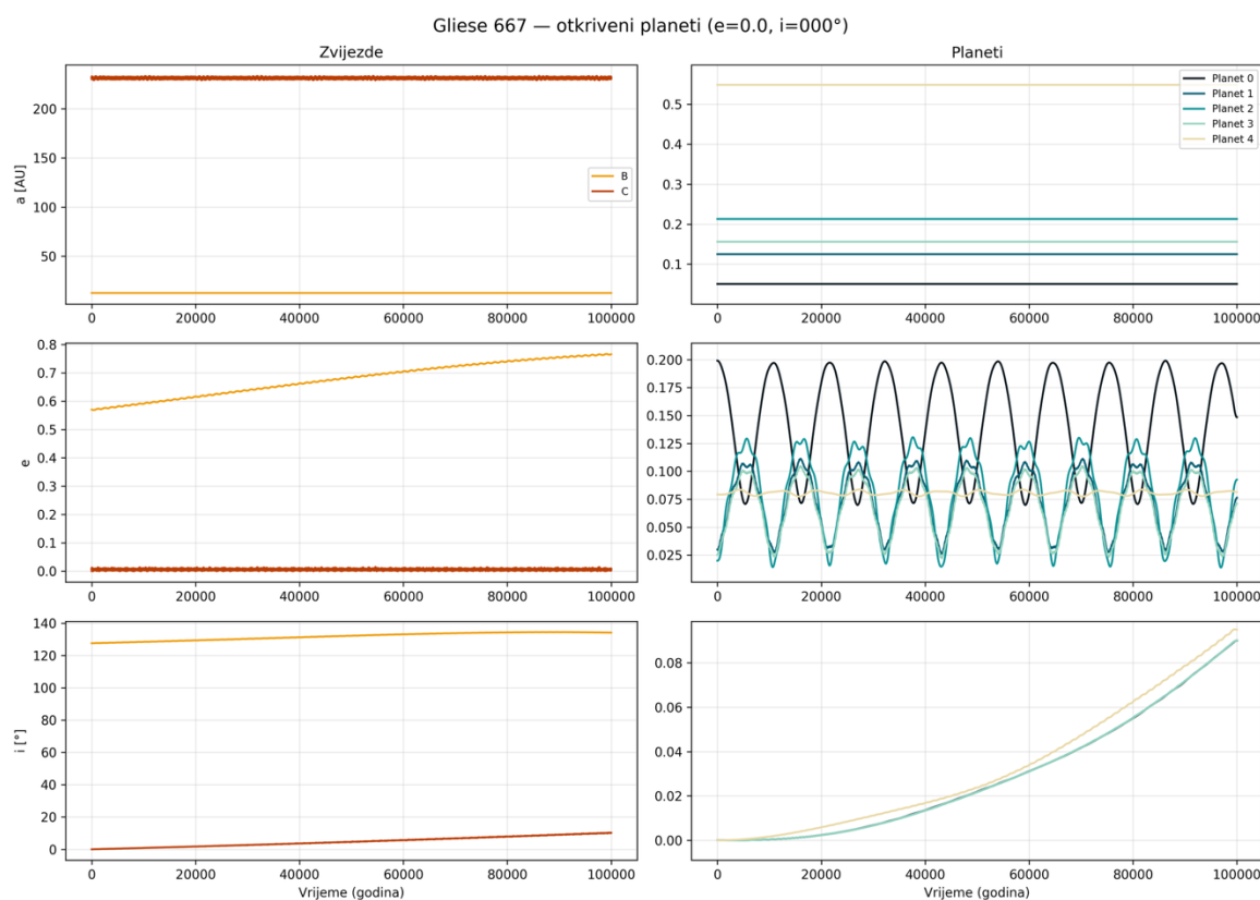
Slika 9: Na lijevoj strani: ovisnost velike poluosi staze, ekscentriciteta i inklinacije zvijezde B i C (crvena boja je zvijezda C, žuta zvijezda B). Na x-osi je vrijeme u godinama. Na desnoj strani: ovisnost velike poluosi staze, ekscentriciteta i inklinacije planeta o vremenu.
