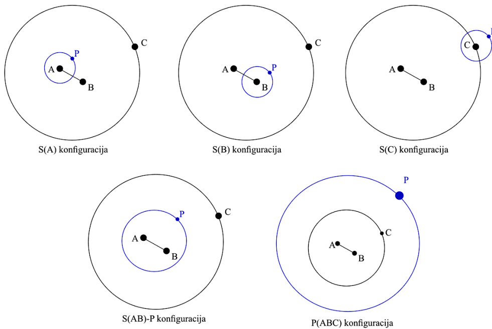
Slika 3: Grafički prikaz 5 jedinstvenih orbitalnih konfiguracija za sustav triju zvijezda i jednog ili više planeta. Ilustracija autora.
