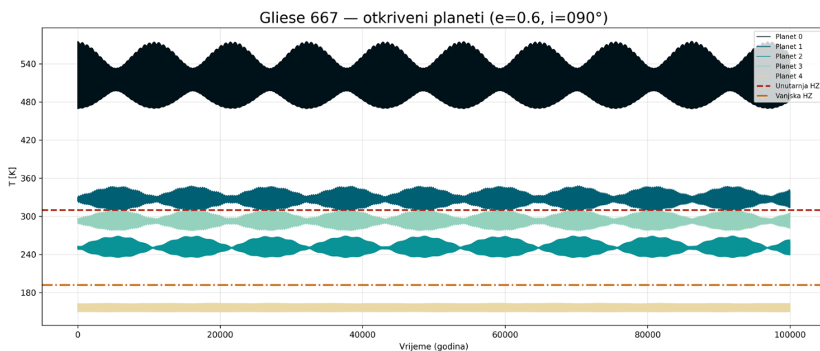
Slika 11: ovisnost temperature o vremenu za planete sustava Gliese 667. Crvena iscrtkana linija označava unutarnju granicu habitabilne zone, a žuta iscrtkana linija vanjsku granicu zone.
