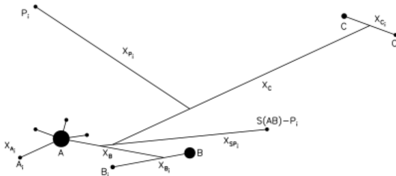
Slika 4: Grafički prikaz koordinatnog sustava za svih 5 konfiguracija. A, B i C su zvijezde, dok P_i su planeti. Linije označavaju udaljenosti od svake komponente konfiguracije, a sjecišta središte mase tih sustava. Ilustracija preuzeta iz [8].
