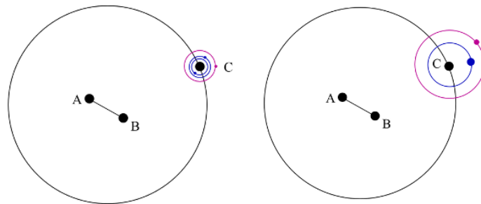
Slika 2: orbitalne konfiguracije sustava LTT 1445 i HD 132563. Plava boja označava stvarne egzoplanete, dok roza boja označava sintetički planet. Ilustracija autora.
