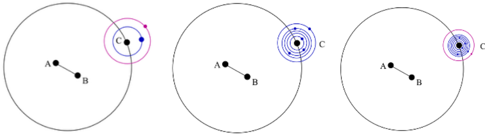
Slika 1: orbitalne konfiguracije sustava 94 Ceti, Gliese 667 i Kepler-444. Plava boja označava stvarne egzoplanete, dok roza boja označava sintetički planet. Ilustracija autora.
