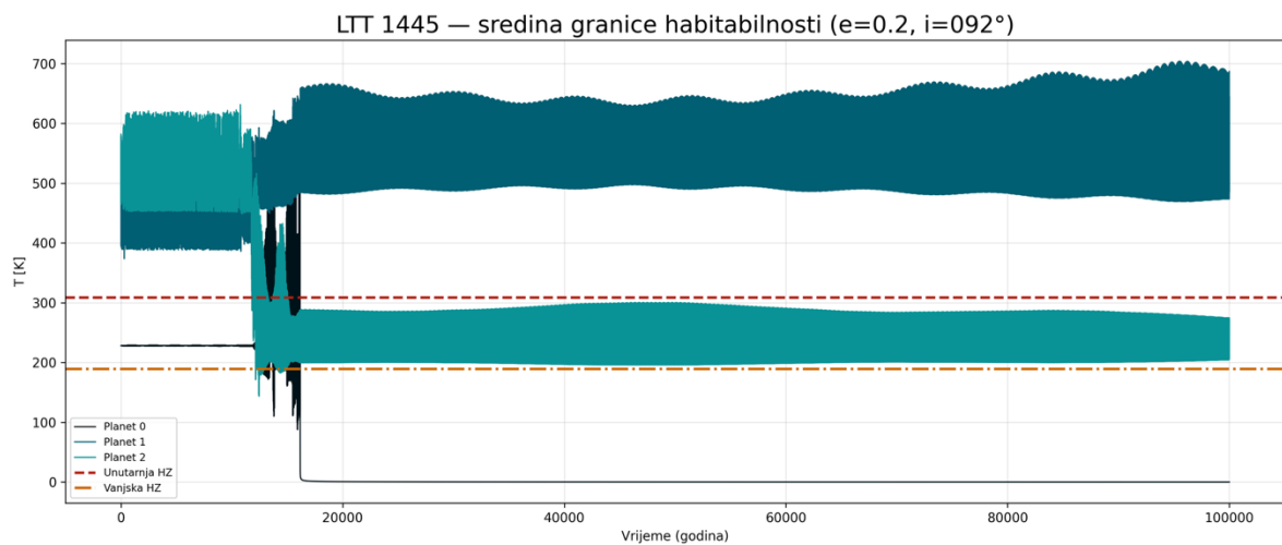
Slika 19: ovisnost temperature o vremenu za planete sustava LTT 1445. Crvena iscrtkana linija označava unutarnju granicu habitabilne zone, a žuta iscrtkana linija vanjsku granicu zone. Nakon što je sintetički planet izbačen iz sustava, drugi planet po redu postaje habitabilan i ostaje u zoni do kraja evolucije.
