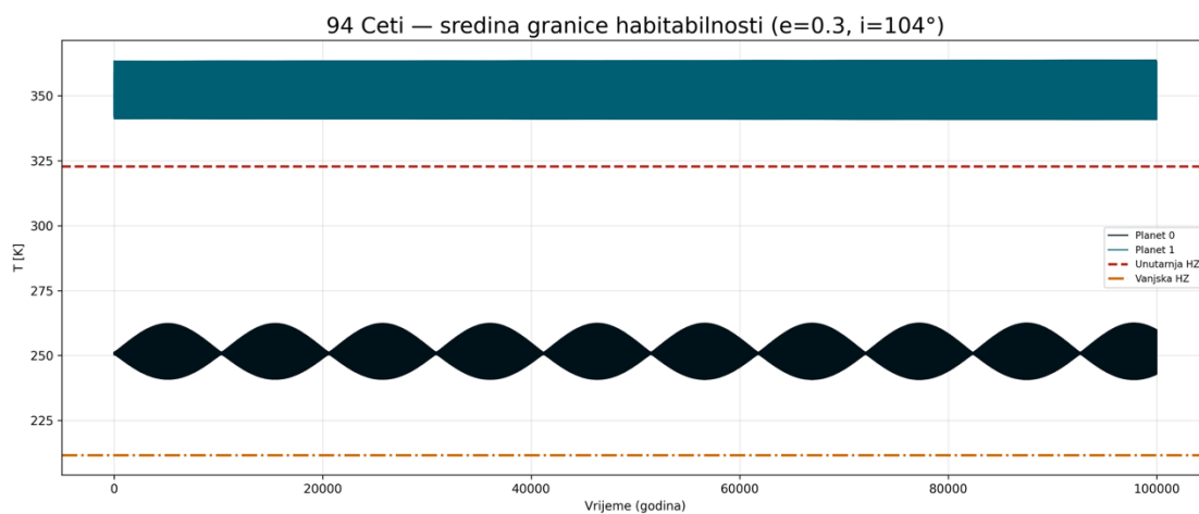
Slika 8: ovisnost temperature o vremenu za planete sustava 94 Ceti. Crna boja označava sintetički planet, a plava stvarni. Crvena iscrtkana linija označava unutarnju granicu habitabilne zone, a žuta iscrtkana linija vanjsku granicu zone.
