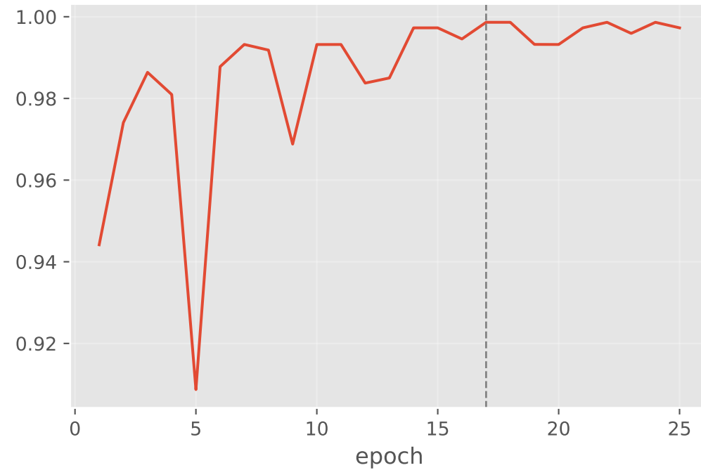
Validation macro-F1
