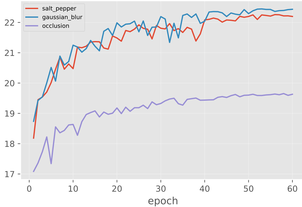
Validation PSNR (dB)
