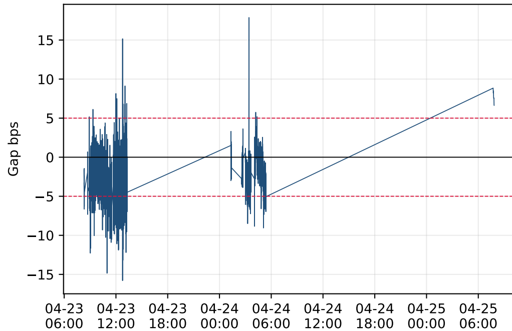
WTI
