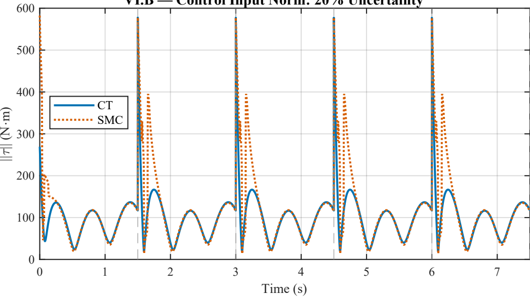
VI.B — Control Input Norm: 20% Uncertainty
