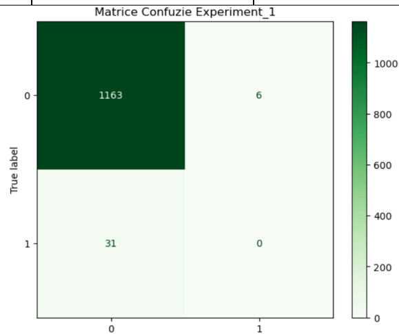
Fig. 3 - Matricea de confuzie exp. 1 Naive Bayes
