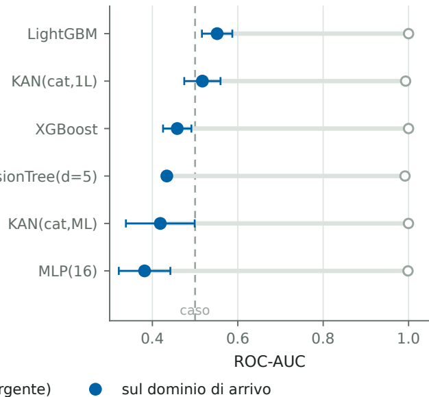
TON→BoT — l'ordinamento è distrutto
