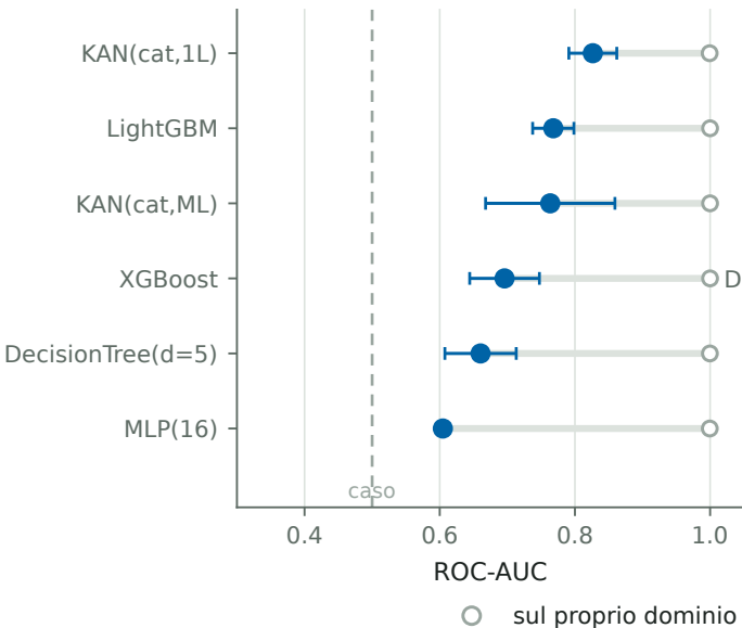
BoT→TON — l'ordinamento regge
